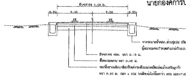
รูปตัดตามแนวตั้งของถนนสายหลัก
