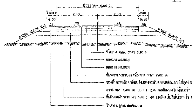
รูปตัดตามแนวตั้งของถนนสายหลัก
