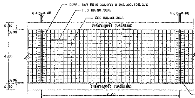
รูปตัดตามแนวตั้งของถนนสายหลัก
