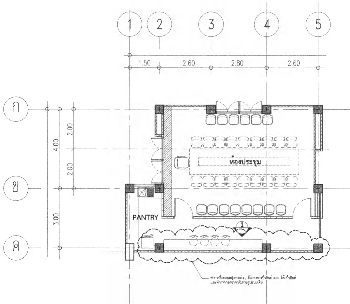
แปลนพื้น -งานรื้อถอน/ปรับปรุง วัดขนาดส่วน 1:75
