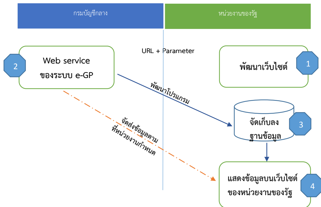
รูปที่ ๒ ขั้นตอนการเชื่อมโยงประกาศจัดซื้อจัดจ้างจากระบบ e-GP ไปยังเว็บไซต์หน่วยงานของรัฐ
