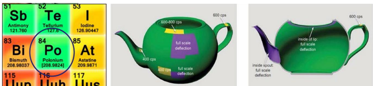
รูปที่ ๓-๖ แสดงวัสดุกัมมันตรังสีส่งผลกระทบภายในร่างกาย
