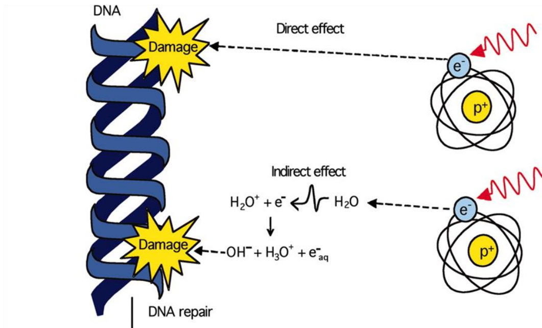
รูปที่ ๒-๘ การทำความเสียหายของรังสีต่อ DNA
