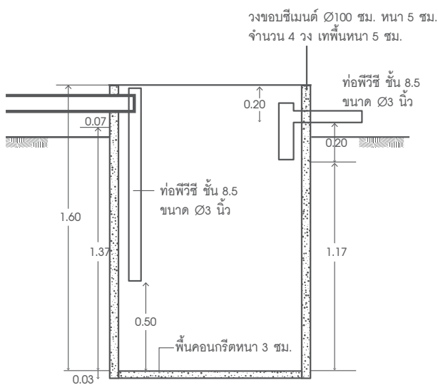
รูปตัดบ่อป๋ม
