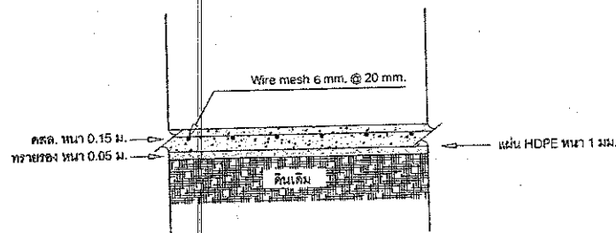
รูปการปิดคลุม (Capping) ด้วยการดาดคอนกรีตหนาประมาณ ๐.๑๕ ม.
