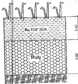
รูปแสดงชั้นการปิดคลุม หนาประมาณ ๑.๐๐ ม. ...”
