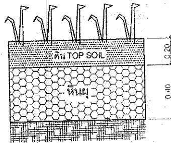
รูปแสดงชั้นการปิดคลุมหนาประมาณ ๐.๖๐ ม.
