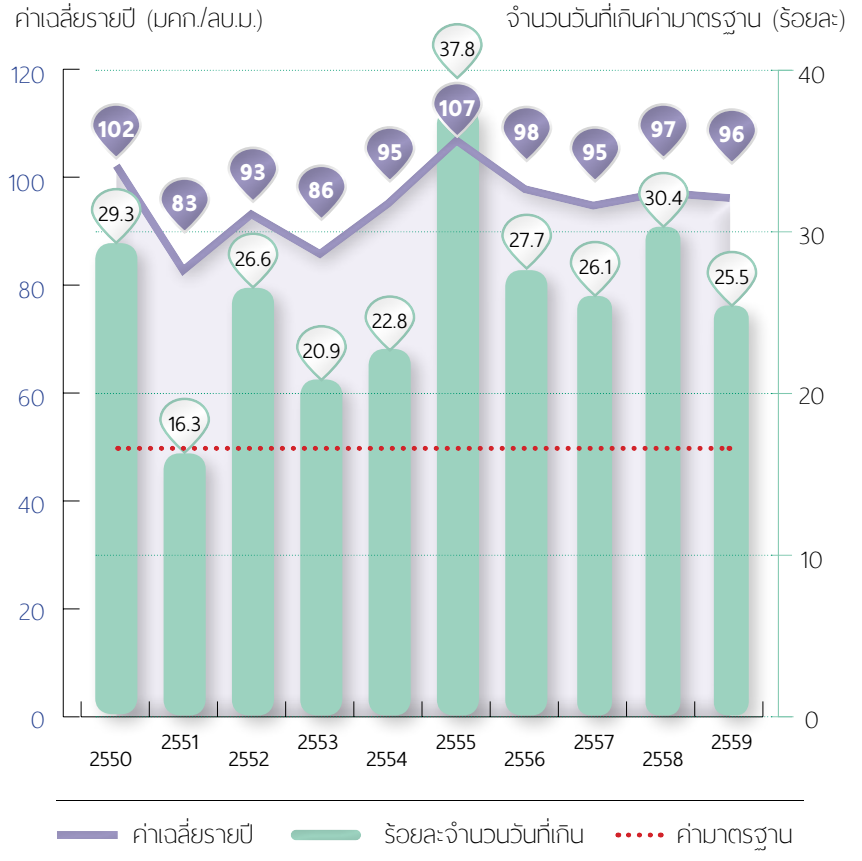
รูปที่ 1-13 สถานการณ์ฝุ่นละออง ( PM_{10} ) ในพื้นที่ตำบลหน้าพระลาน อำเภอเฉลิมพระเกียรติ จังหวัดสระบุรี
