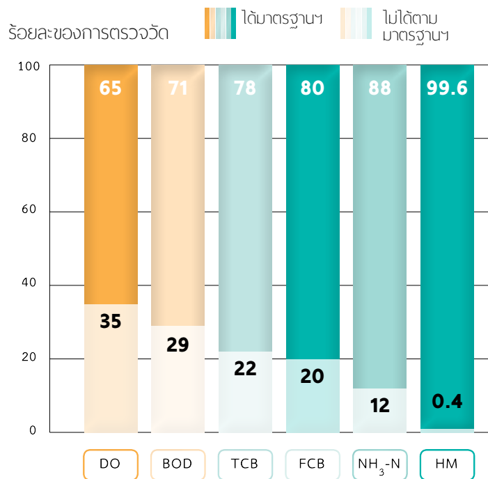
รูปที่ 2-3 ผลการตรวจวัดคุณภาพน้ำในภาคกลางเทียบกับมาตรฐานคุณภาพน้ำในแหล่งน้ำผิวดินประเภทที่ 3
