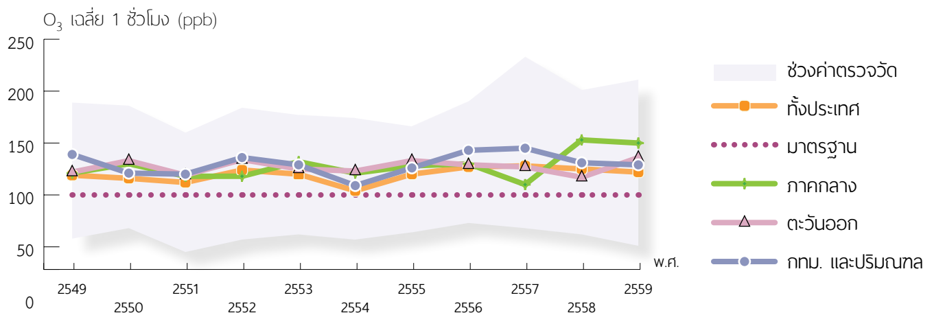
รูปที่ 1-4 ผลการตรวจวัดก๊าซโอโซน ค่าเฉลี่ย 1 ชั่วโมงสูงสุดของปี เฉลี่ยรายพื้นที่ ปี 2549-2559 เปรียบเทียบพื้นที่ที่พบก๊าซโอโซนปริมาณสูง
