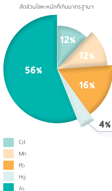
รูปที่ 2-2 ผลการตรวจวัดคุณภาพน้ำในภาคเหนือ เทียบกับมาตรฐานคุณภาพน้ำ ในแหล่งน้ำผิวดินประเภทที่ 3
