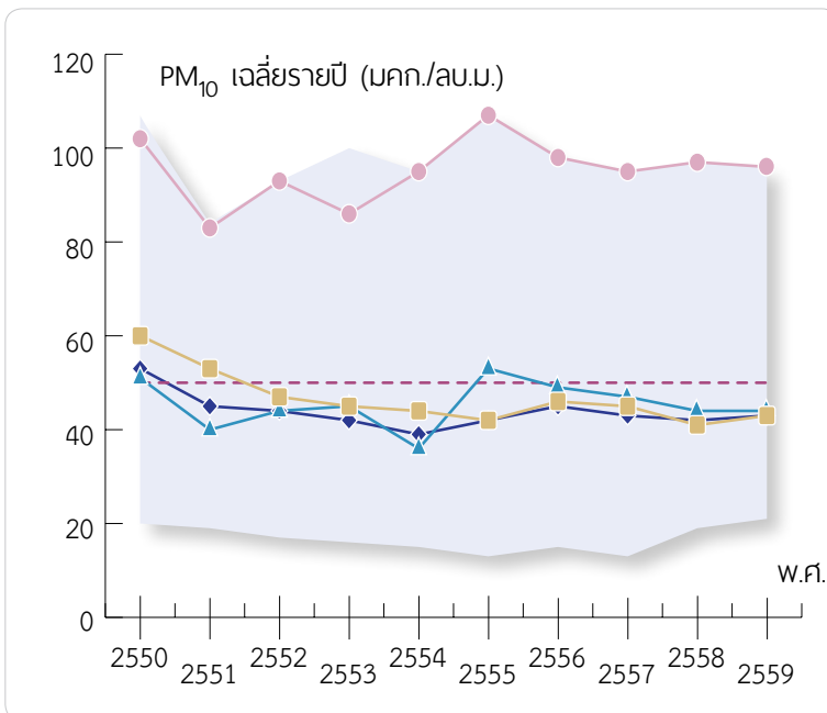
รูปที่ 1-1 ความเข้มข้นฝุ่นละออง ( PM_{10} ) ในบรรยากาศ เฉลี่ยรายปี เฉลี่ยรายพื้นที่ ปี 2550-2559
