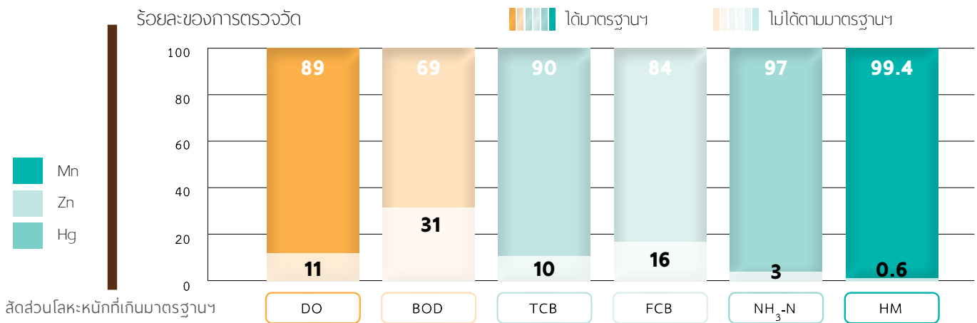
รูปที่ 2-6 ผลการตรวจวัดคุณภาพน้ำในภาคใต้เทียบกับมาตรฐานคุณภาพน้ำในแหล่งน้ำผิวดินประเภทที่ 3
