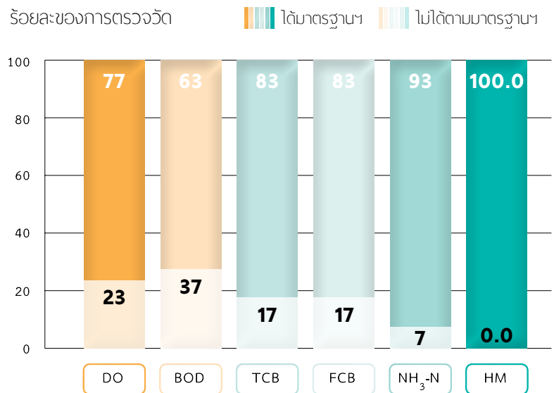
รูปที่ 2-5 ผลการตรวจวัดคุณภาพน้ำในภาคตะวันออกเทียบกับมาตรฐานคุณภาพน้ำในแหล่งน้ำผิวดินประเภทที่ 3
