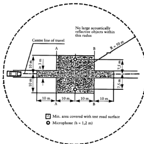
รูปที่ ๑ คุณลักษณะขั้นต่ำสำหรับบริเวณพื้นผิวทดสอบ ส่วนที่แรงแสดงพื้นที่ทดสอบ
