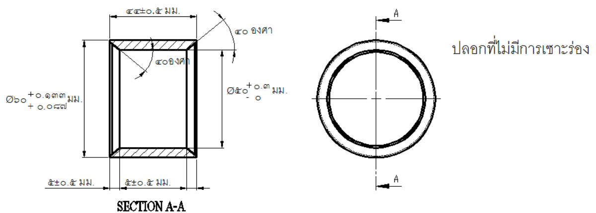
รูปที่ ๑๓ ปลอกที่ไม่มีการเจาะรู
