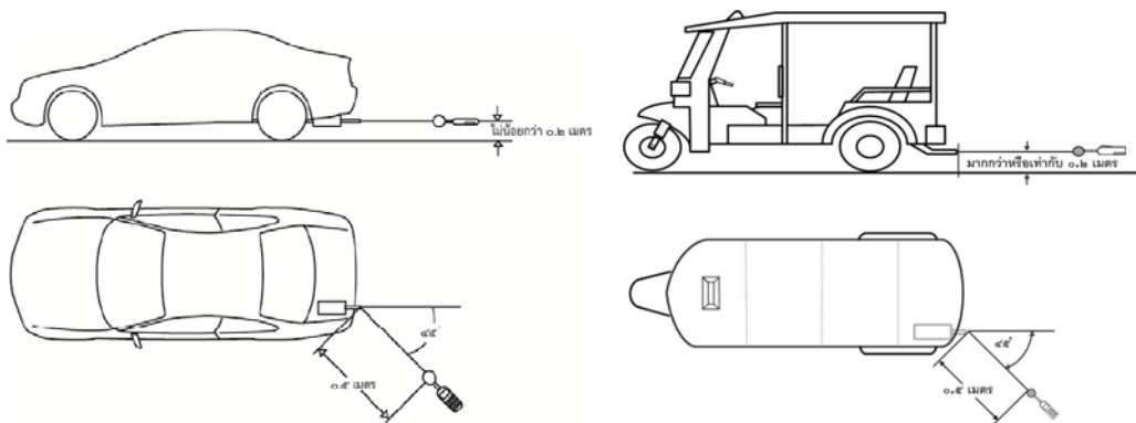
ภาพที่ ๒ ตำแหน่งการตั้งไมโครโฟนของมาตรฐานระดับเสียง กรณีรถยนต์มีปลายท่อไอเสียท่อเดียว และยื่นพ้นริมนอกสุดของตัวถังรถ
