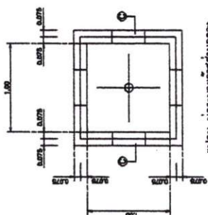
แปลน บ่อระบายน้ำส่วนกลาง
