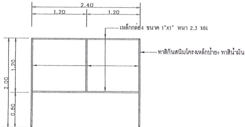
แบบโครงหลัก มาตราส่วน 1:100
