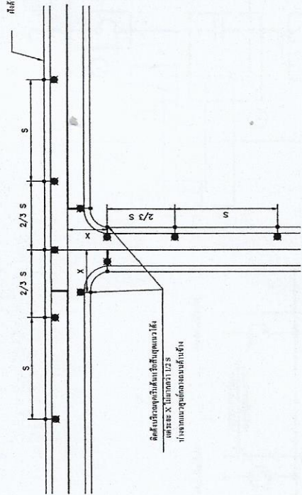
รูปแบบการติดตั้งเสาไฟฟ้าส่องสว่างบนบริเวณสามแยก
