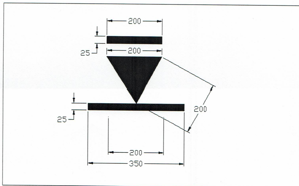
รูปที่ ๒ แสดงเครื่องหมายแนวน้ำบรรทุกสำหรับเรือลำน้ำที่มีใช้เรือกล
