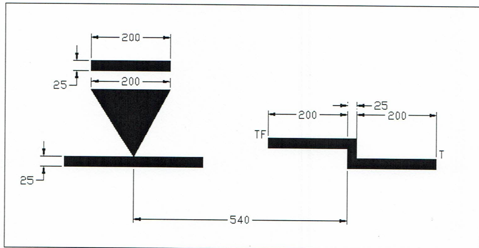
รูปที่ ๒ แสดงเครื่องหมายแนวน้ำบรรทุกสำหรับเรือลำน้ำที่มีใช้เรือกล
