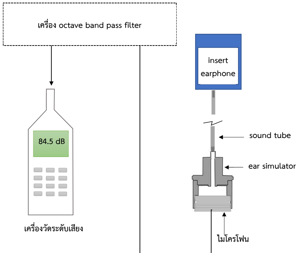
รูปที่ 3 การต่ออุปกรณ์สำหรับการวัดระดับความดันเสียงและการควบคุมระดับสัญญาณ
