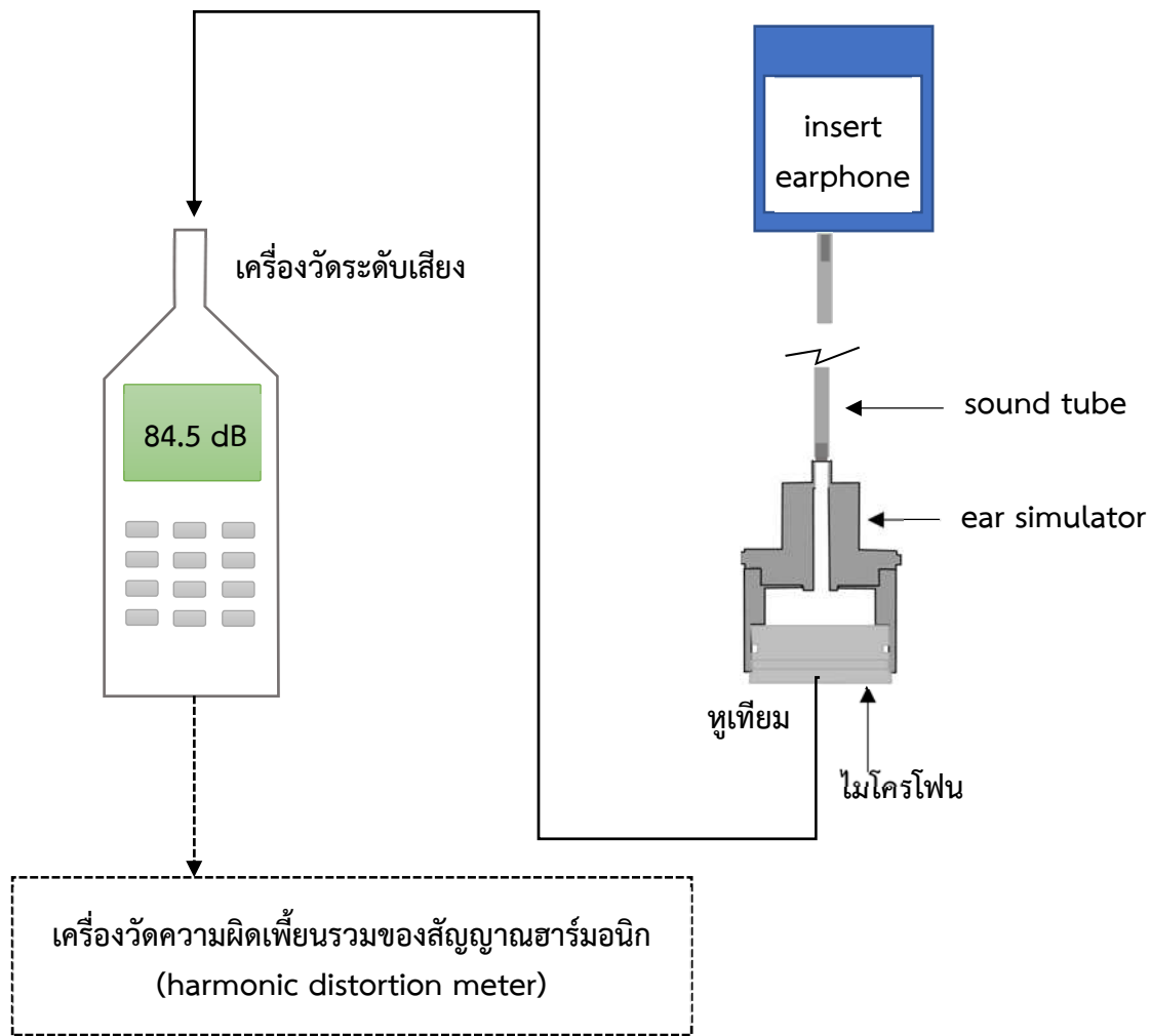
รูปที่ 5 แสดงการต่ออุปกรณ์สำหรับการวัดค่าความผิดเพี้ยนรวมของสัญญาณฮาร์มอนิกของสัญญาณเสียง
