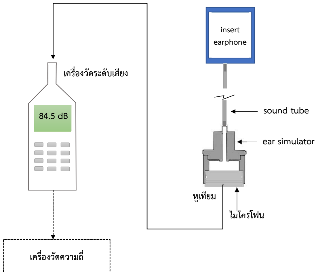
รูปที่ 2 แสดงการต่ออุปกรณ์สำหรับการวัดความถี่
