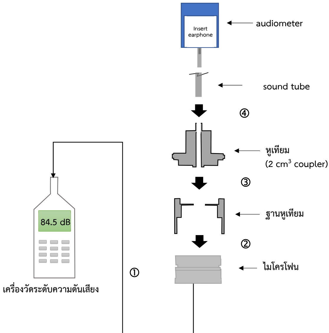
รูปที่ 1 แสดงการประกอบหูเทียมและเครื่องวัดระดับเสียง
