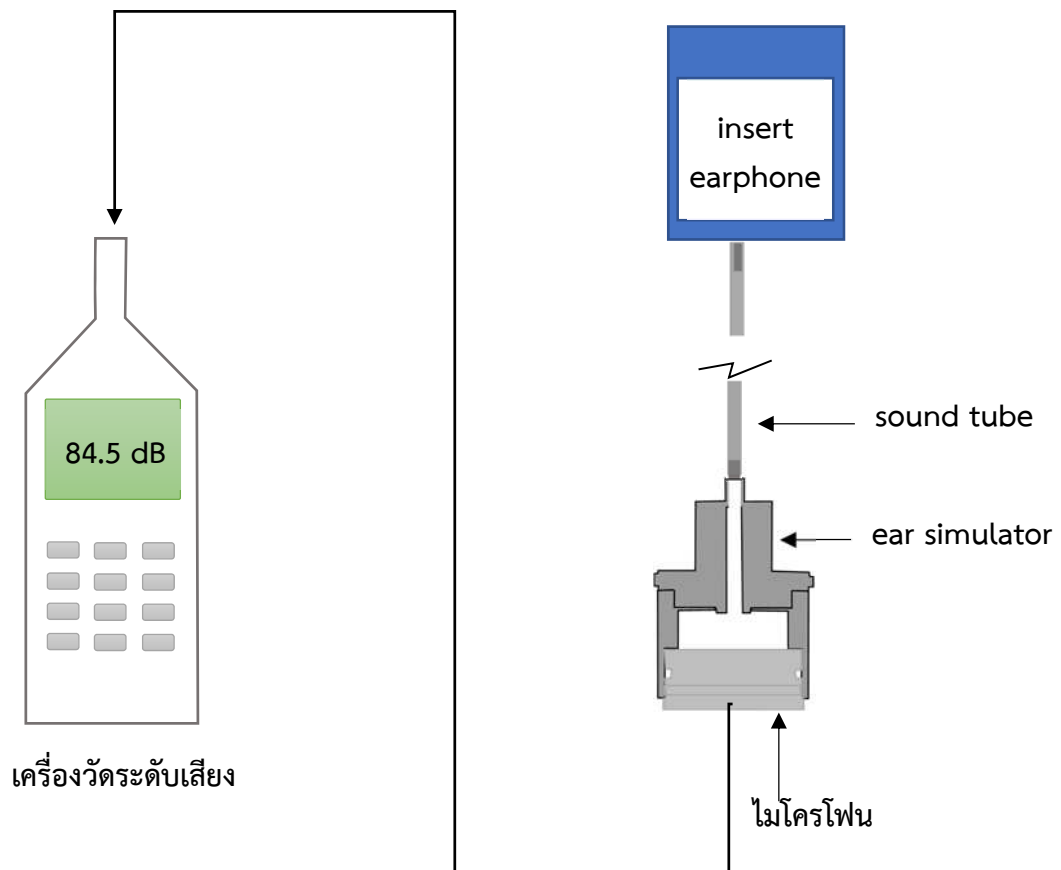
รูปที่ 4 แสดงการต่ออุปกรณ์สำหรับการวัดระดับเสียงลง (masking noise level)
