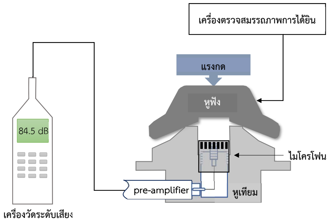
รูปที่ 4 แสดงการต่ออุปกรณ์สำหรับการวัดระดับเสียงลง
