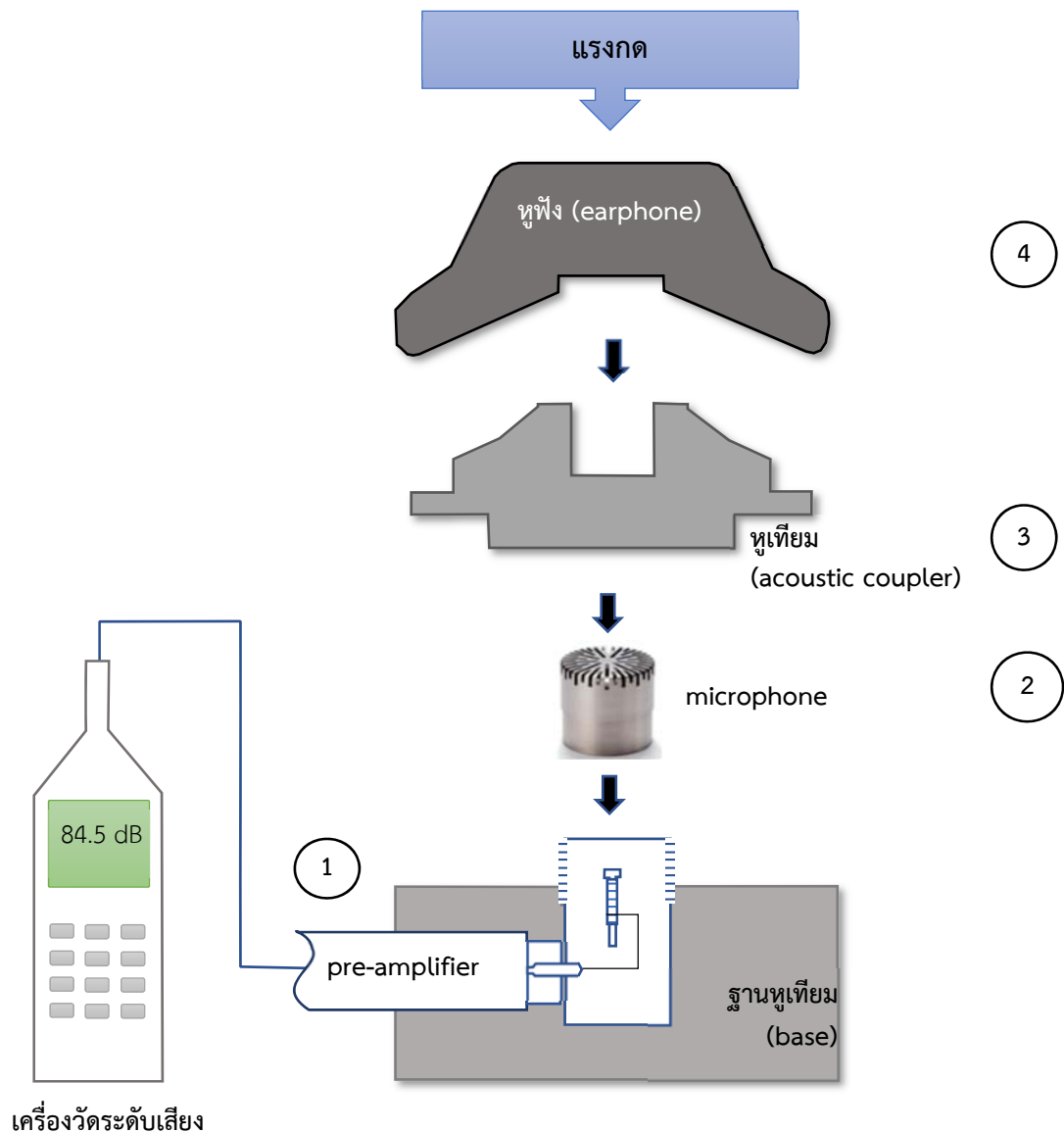
รูปที่ 1 แสดงการประกอบหูเทียมและเครื่องวัดระดับเสียง
