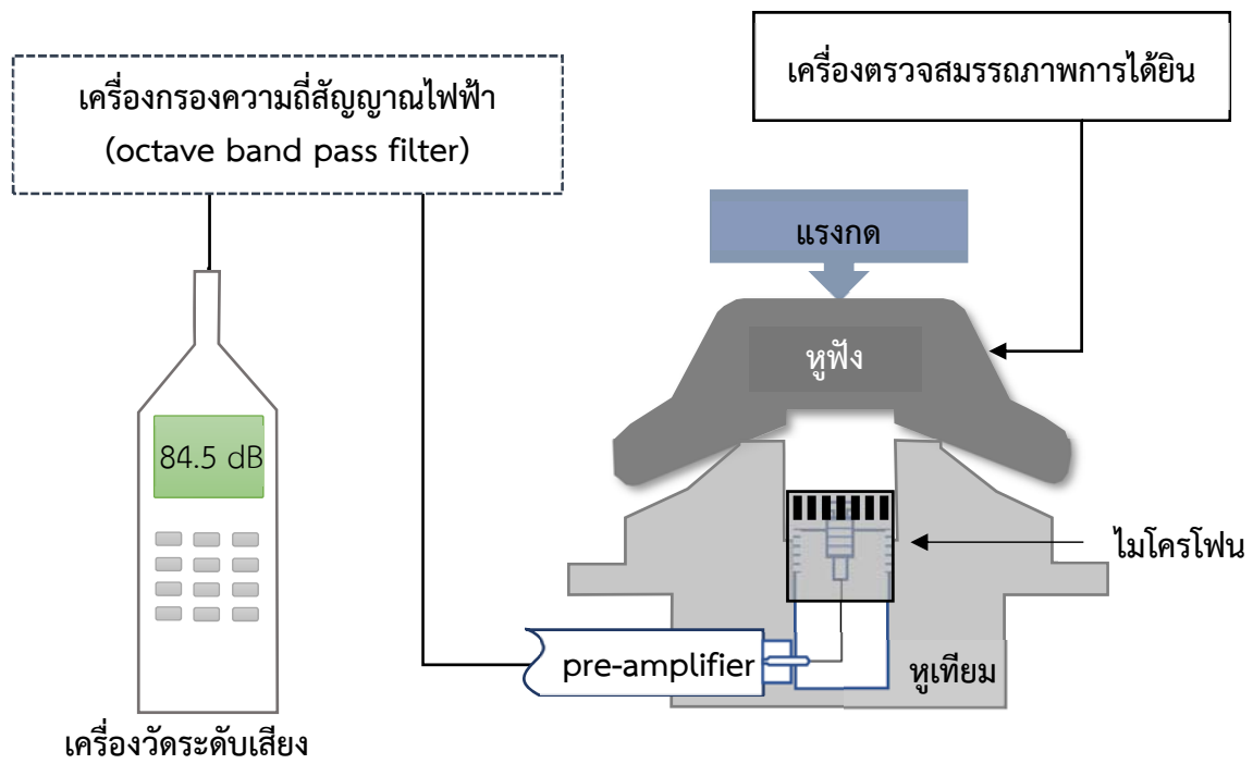
รูปที่ 3 การต่ออุปกรณ์สำหรับการวัดระดับความดันเสียงและการควบคุมระดับสัญญาณ
