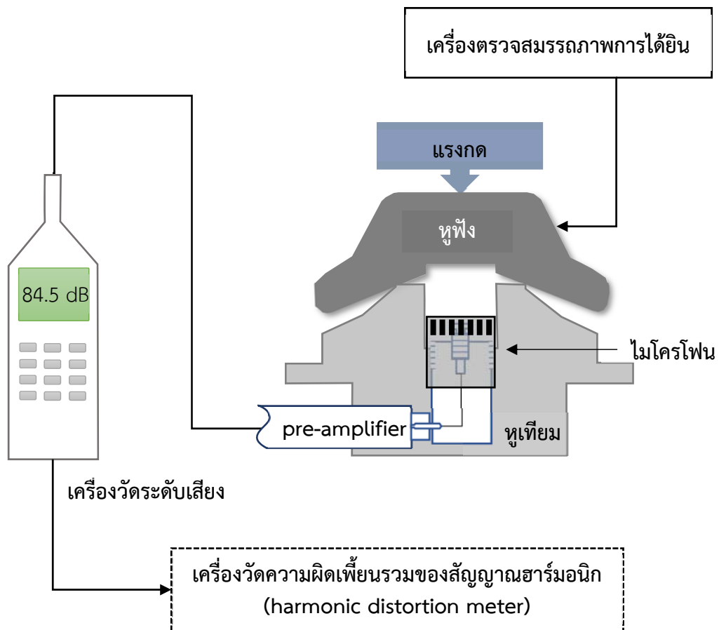
รูปที่ 5 แสดงการต่ออุปกรณ์สำหรับการวัดค่าความผิดเพี้ยนรวมของสัญญาณฮาร์มอนิก
