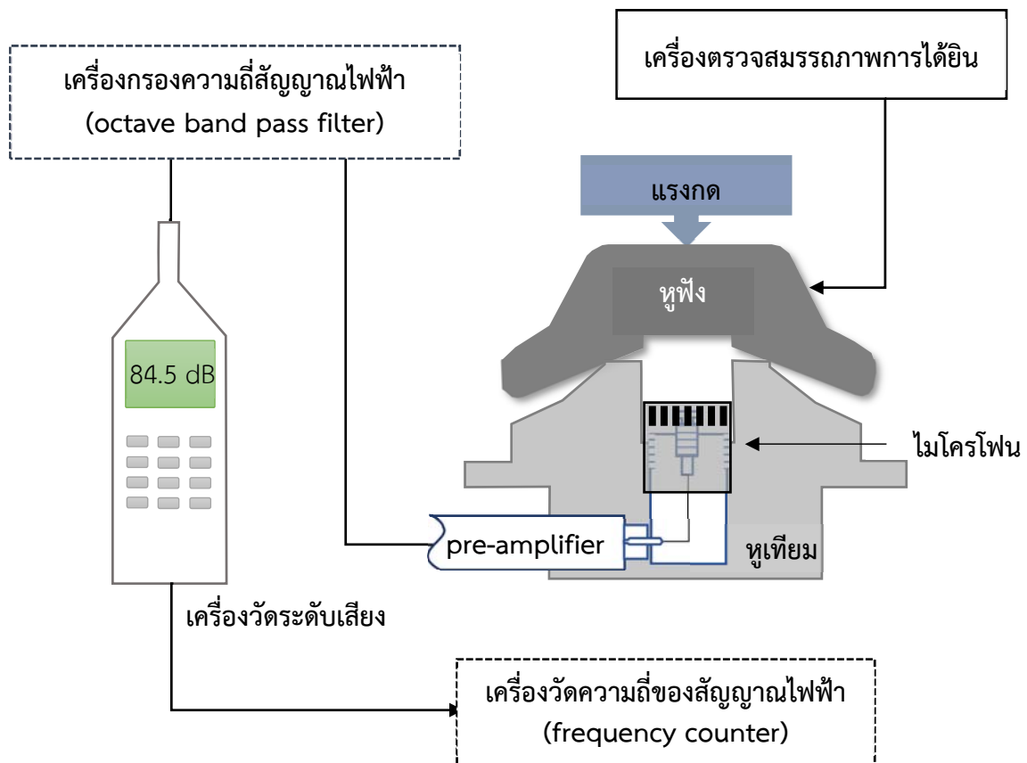
รูปที่ 2 แสดงการต่ออุปกรณ์สำหรับการวัดความถี่
