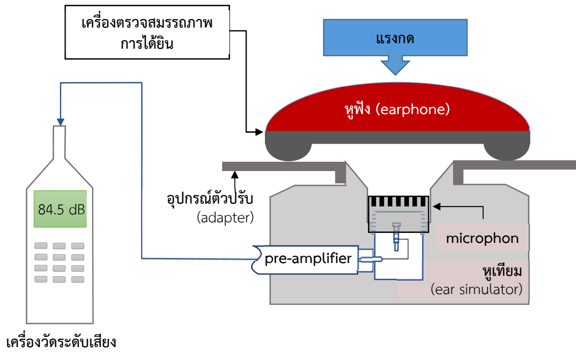
รูปที่ 4 แสดงการต่ออุปกรณ์สำหรับการวัดระดับเสียงลง
