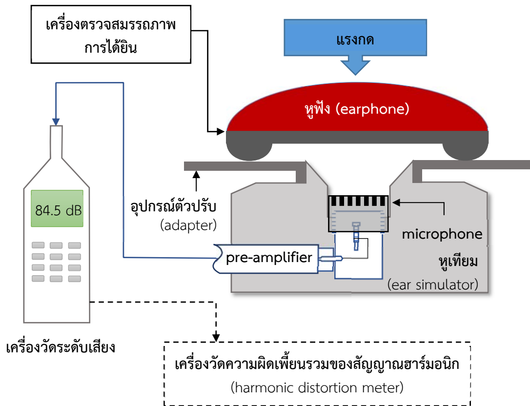
รูปที่ 5 แสดงการต่ออุปกรณ์สำหรับการวัดค่าความผิดเพี้ยนรวมของสัญญาณเสียง
