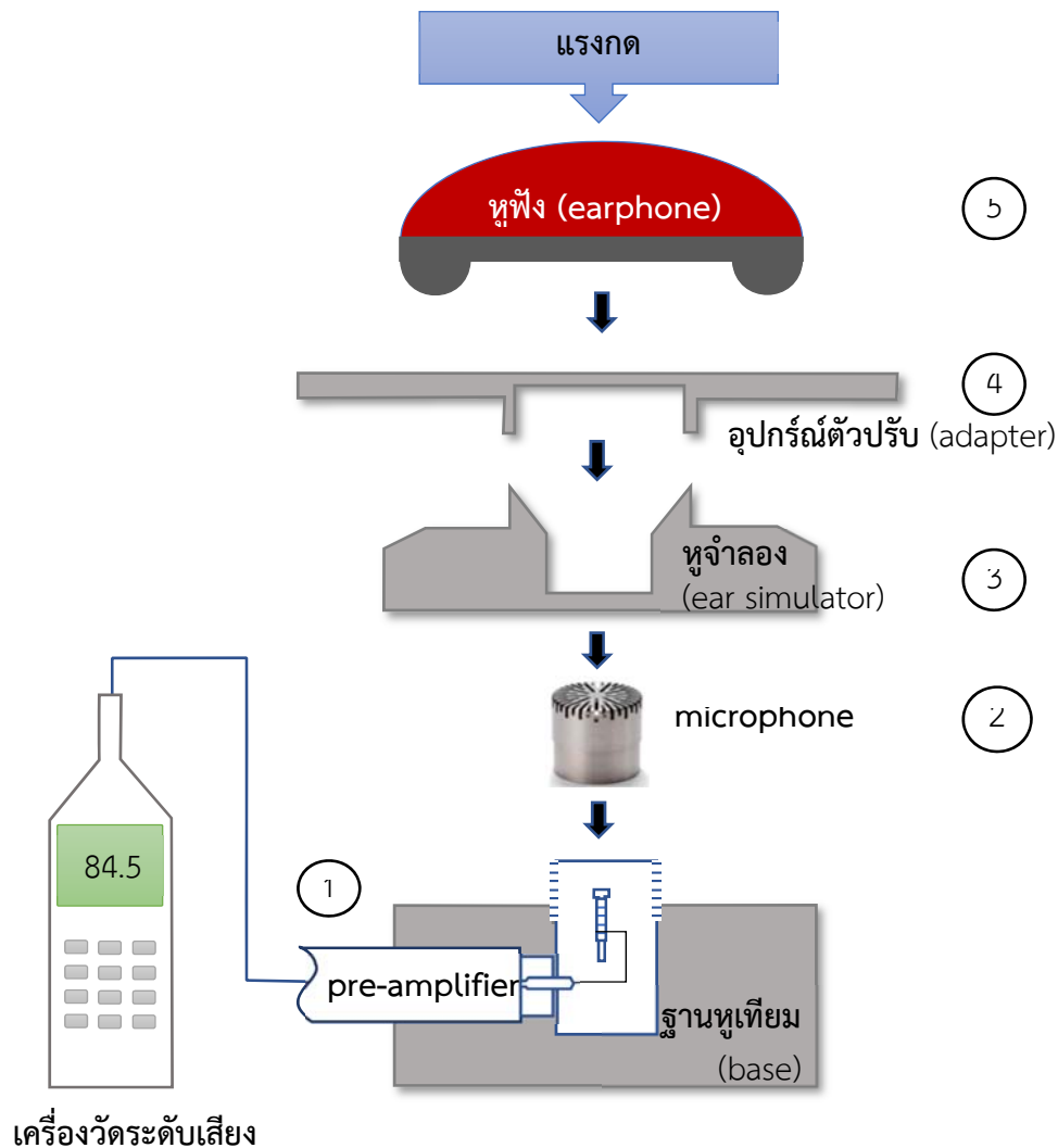
รูปที่ 1 แสดงการประกอบหูเทียมและเครื่องวัดระดับเสียง
