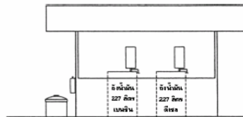
รูปที่ 4-7 รูปด้านท้ายถังน้ำมันฐานสกีขนาดบรรจุไม่เกิน 9,600 ลิตร
