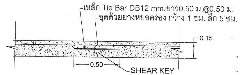
LONGITUDINAL JOINT
