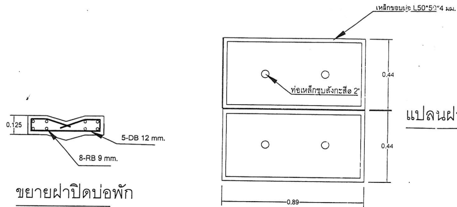
รูปตัดฝาบ่อพัก
