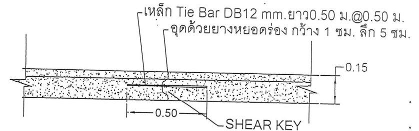
LONGITUDINAL JOINT
