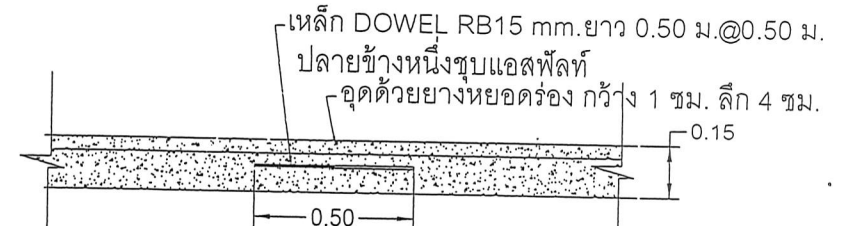
CONTRACTION JOINT ทุกๆระยะไม่เกิน 10 ม.
