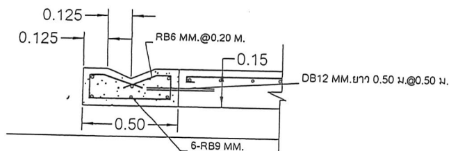
ขยายร่างวิ คสล.
