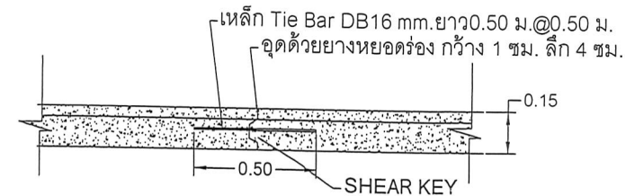
LONGITUDINAL JOINT
