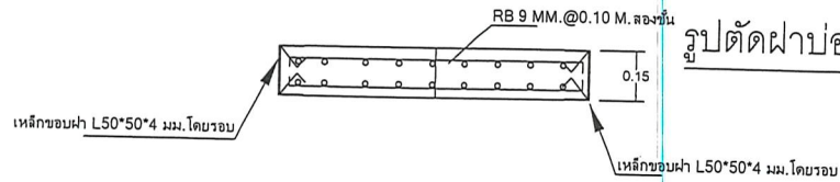
ขยายฝาปิดบ่อพัก
