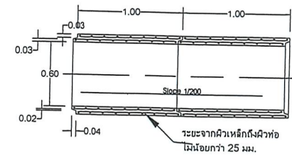
รูปตัดท่อระบายน้ำ คสล.
