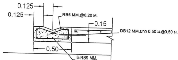
ขยายรางวิค.ส.ล.
