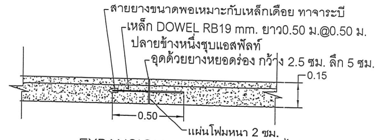
EXPANSION JOINT ทุกๆระยะไม่เกิน 30 ม.
