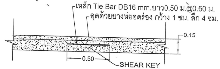
LONGITUDINAL JOINT
