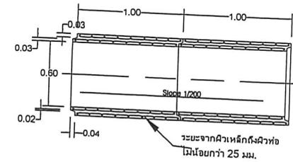
รูปตัดท่อระบายน้ำ คสล.
