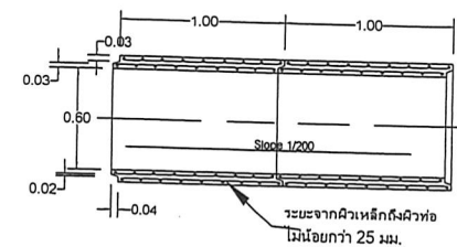
รูปตัดท่อนระบายน้ำ คสล.
