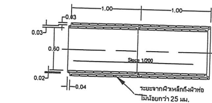
รูปตัดท่อระบายน้ำ คสล.
