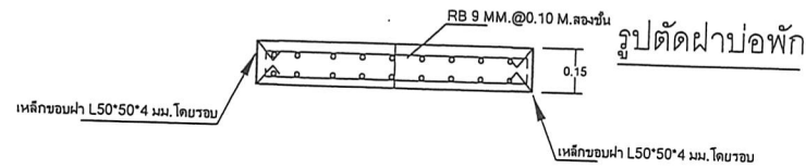
ขยายฝาปิดบ่อพัก
