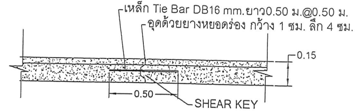
LONGITUDINAL JOINT
