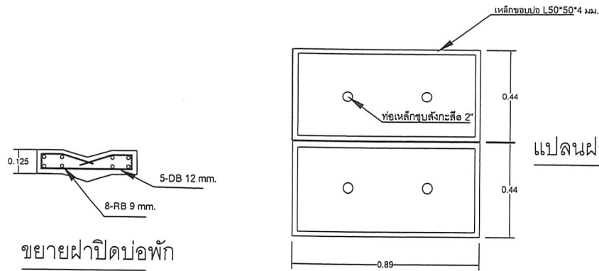
รูปตัดฝาปิด
