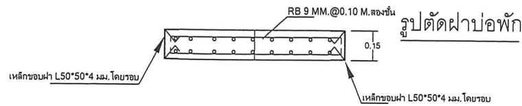
ขยายฝาปิดบ่อพัก
