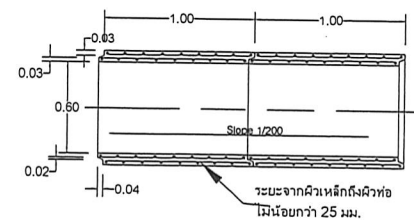
รูปตัดท่อนระบายน้ำ คสล.
