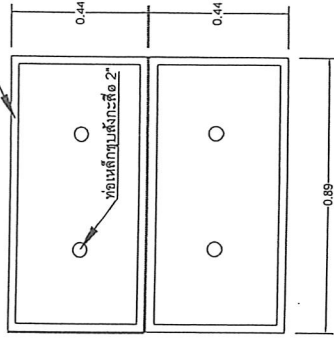
แปลนฝาปิด
