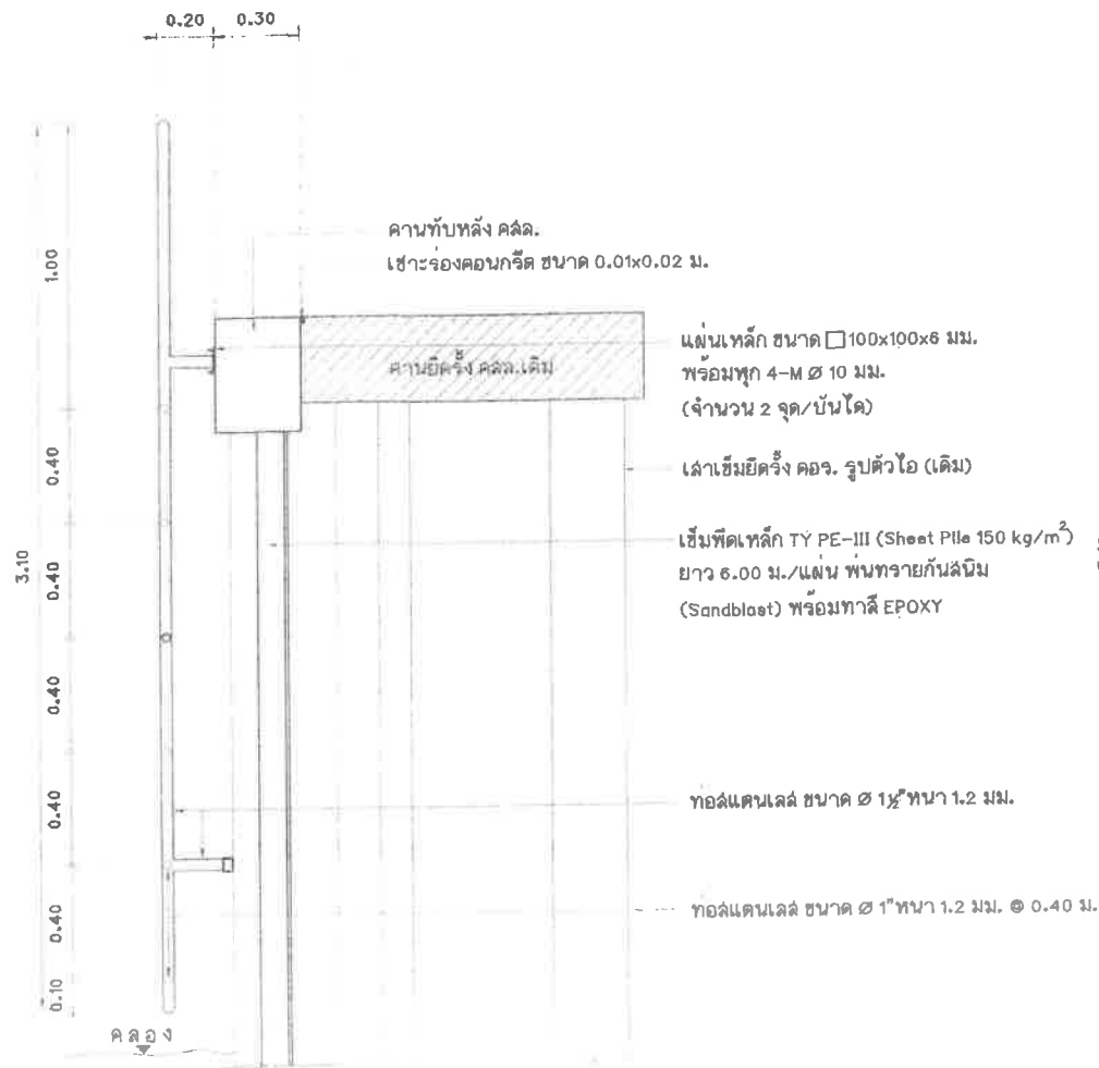
รูปตัด ด้านข้างบันไดลงถัง มาตราส่วน 1:20
