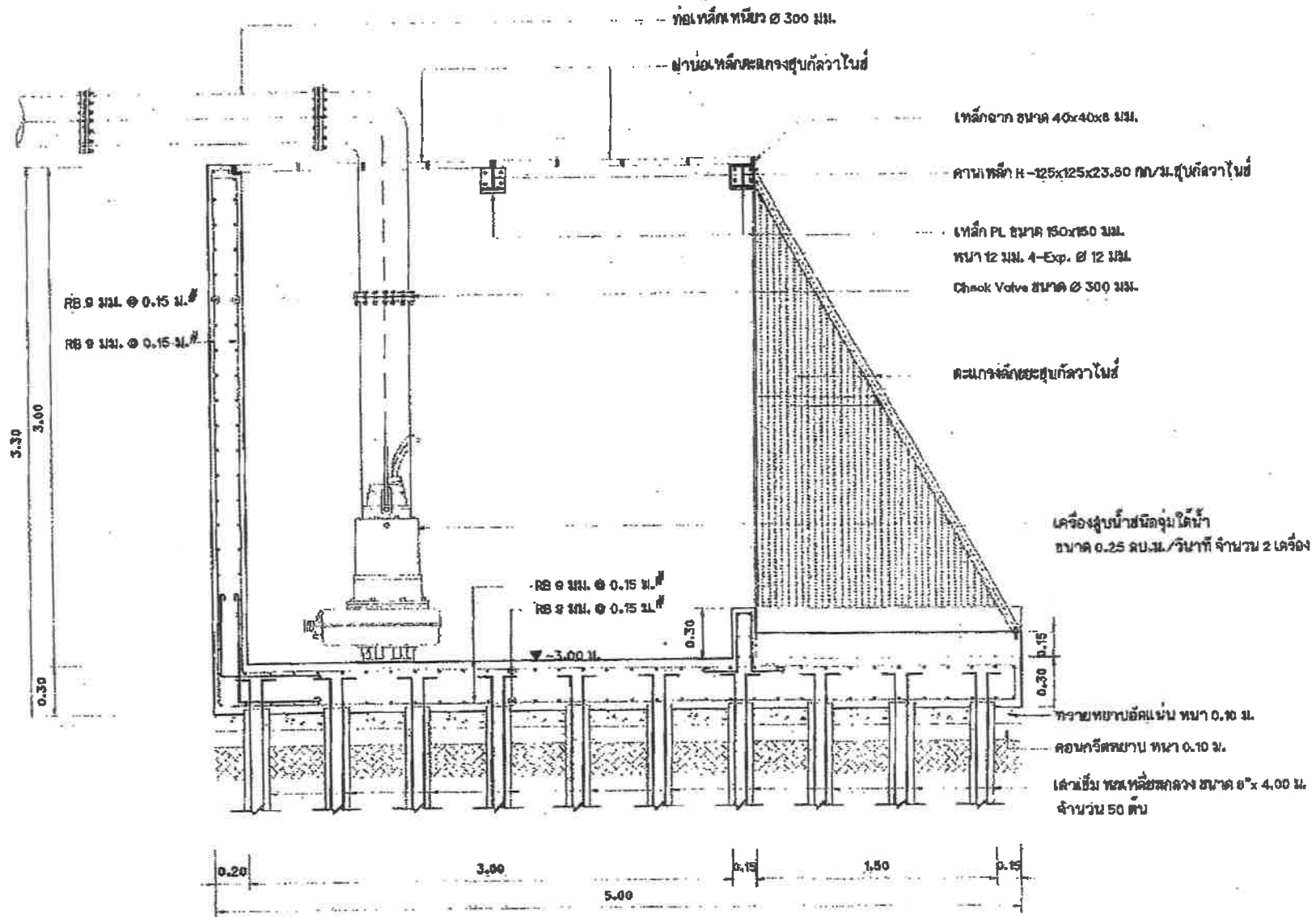
รูปตัดโครงสร้าง ๑ บ่อสูบน้ำ คลล.
