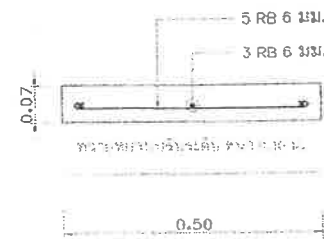
แบบขยายรูปตัดแปลนพื้นร่องท่อ มาตราส่วน 1 : 10
