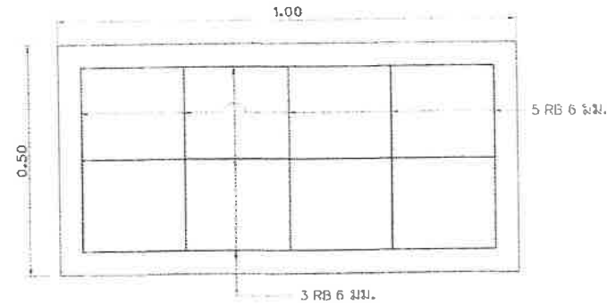
แบบขยายแปลนพื้นร่องท่อ มาตราส่วน 1 : 10
