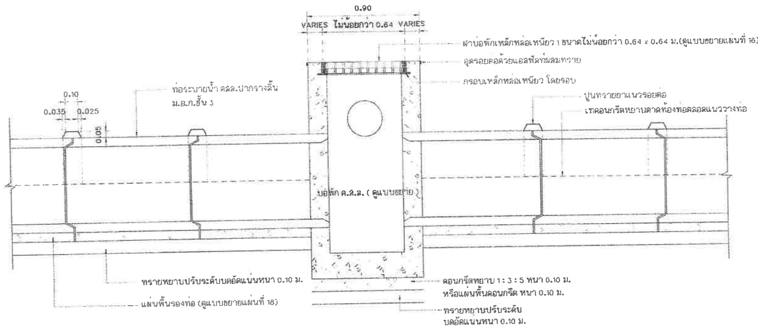
รูปตัดตามยาวการวางทอร์บายน้ำ มาตราส่วน 1 : 20
