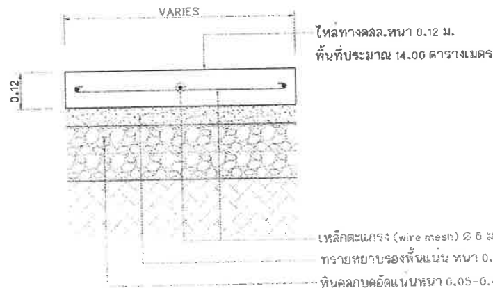
แบบขยายรูปตัดทางเข้าบ้าน คสล.หนา 0.12 ม. มาตราส่วน 1 : 10
