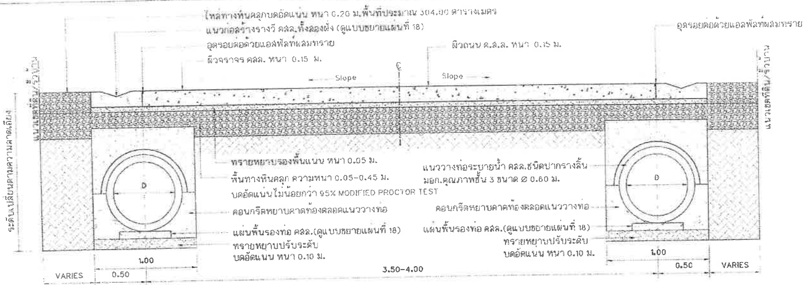
แบบขยายรูปตัด 1 (แบบมีไหล่ทางหินคลุก) มาตราส่วน 1:25
