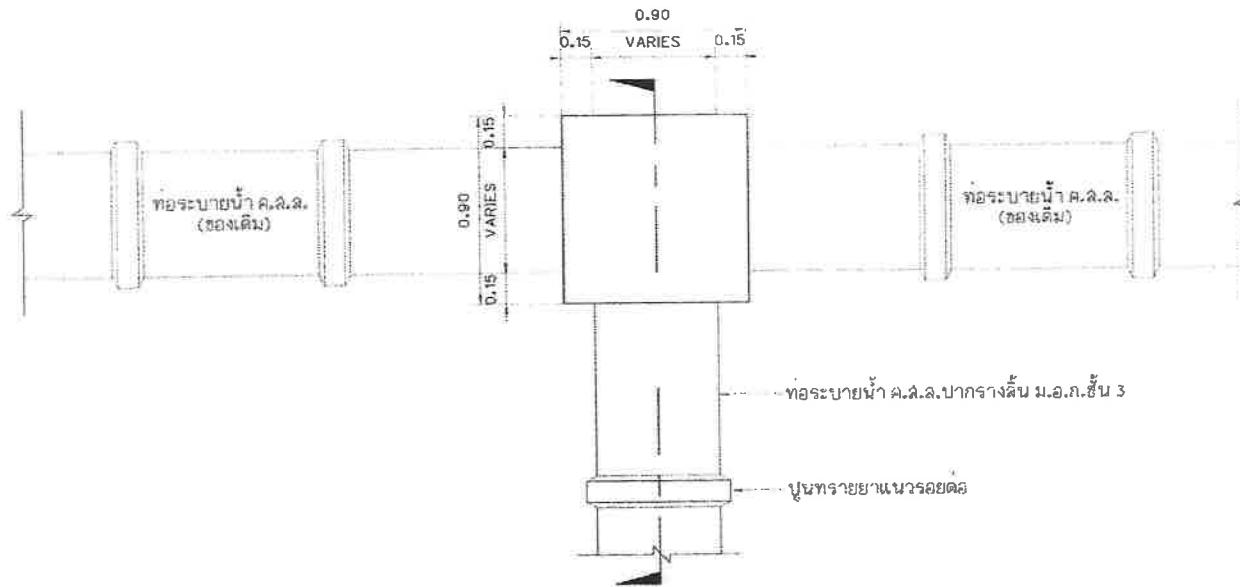
แบบแผนการเชื่อมต่อในกรณีเชื่อมกับท่อน้ำประปาของเดิม มาตราส่วน 1:25
