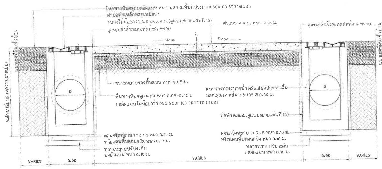
แบบขยายรูปตัด 2 (แบบมีไหล่ทางหินคลุก) มาตราส่วน 1:25
