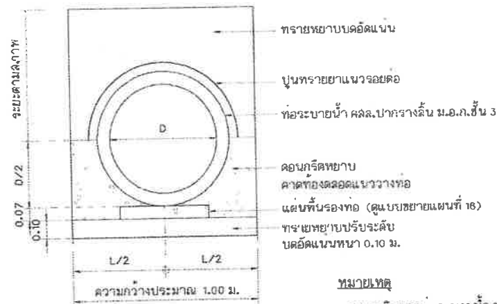
แบบขยายการวางท่อระบายน้ำ คลล. มาตราส่วน 1 : 20
