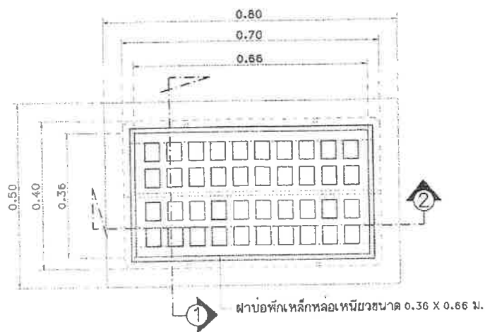
แบบขยายฝาบ่อพักรางวล์เหล็กหล่อเหนียว มาตราส่วน 1 : 10
