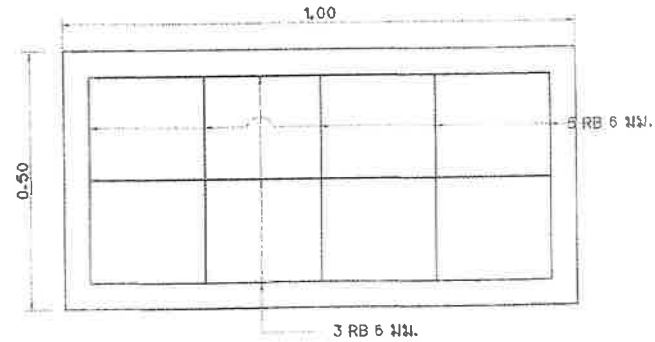
แบบขยายแปลนแผ่นพื้นรองทอ มาตราส่วน 1 : 10
