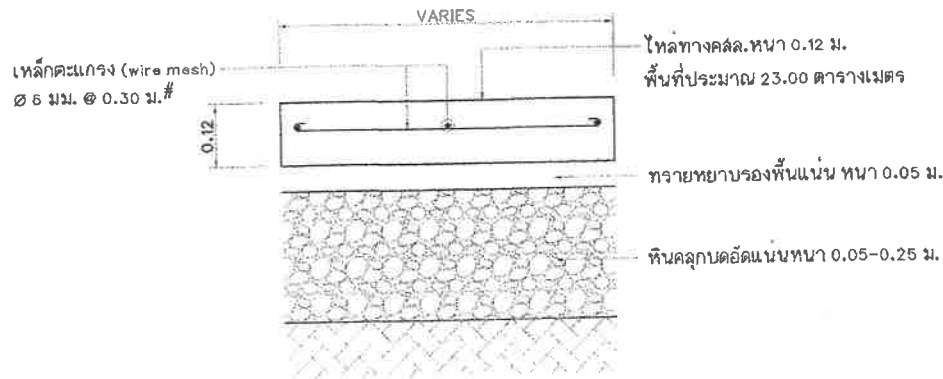
แบบขยายรูปตัดทางเข้าบ้าน คสล.หนา 0.12 ม. มาตราส่วน 1 : 10
