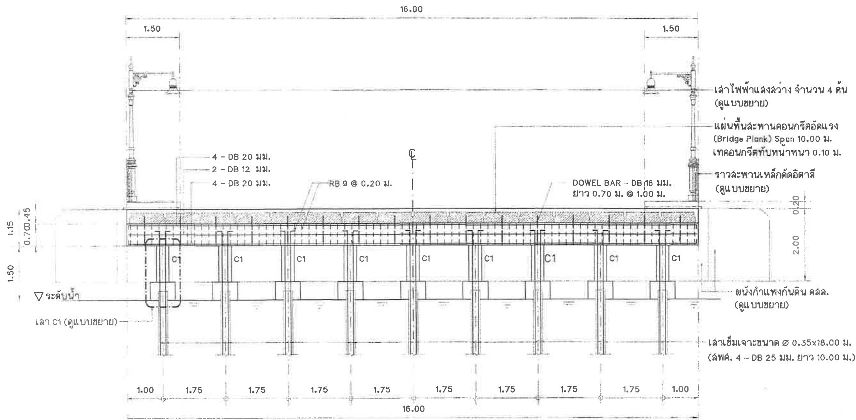
รูปตัดโครงสร้างสะพาน A - A มาตราส่วน 1:75
