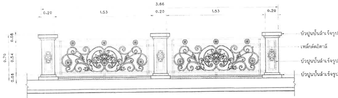
แบบขยายรูปด้านหน้าราวสะพานเหล็กดัดอิตาลี มาตราส่วน 1:20
