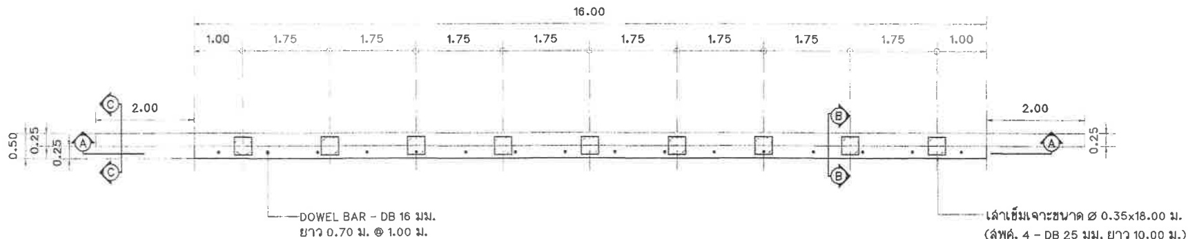
ขยายโครงสร้างสะพาน มาตราส่วน 1:75
