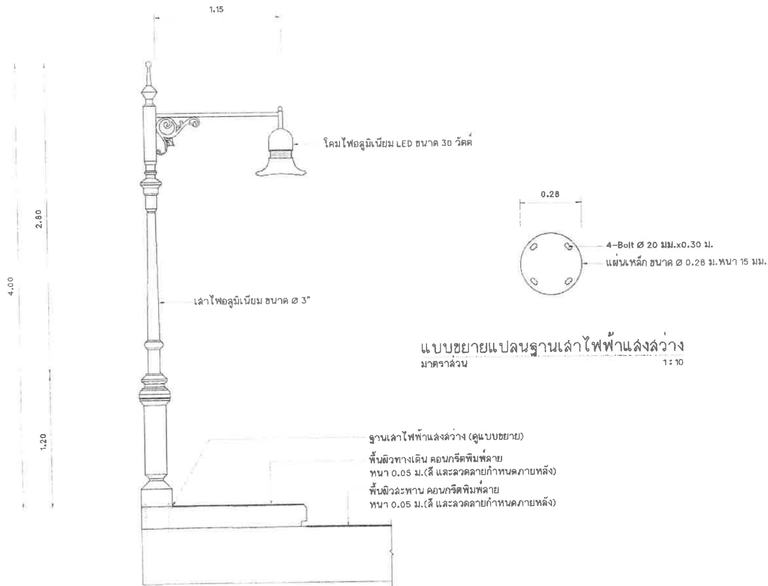
แบบขยายเสาไฟฟ้าแสงสว่าง มาตราส่วน 1 : 25
