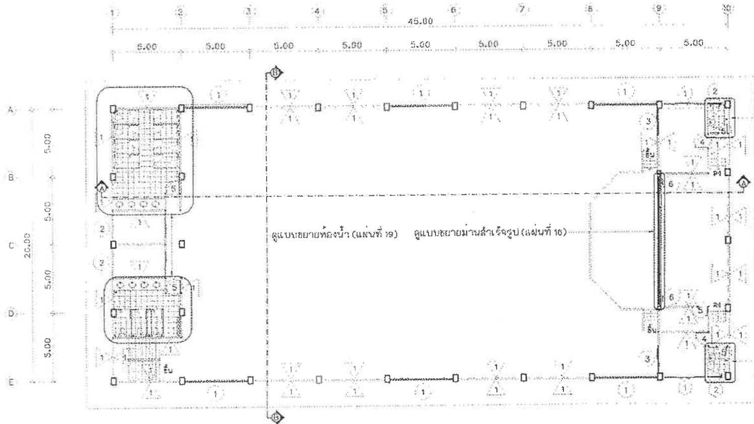
แปลนพื้นที่ชั้นล่างที่ปรับปรุง มาตรฐาน 1: 200
