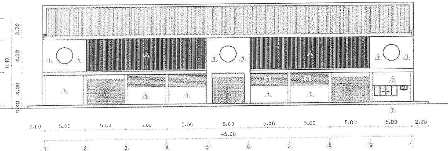
รูปด้าน 3 ที่ปรับปรุง มาตราส่วน 1:200
