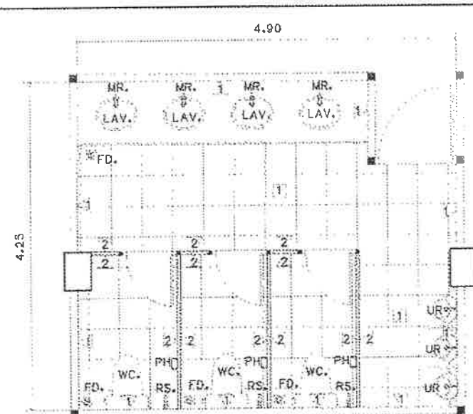
แบบขยายห้องน้ำ มาตรฐาน 1:50
