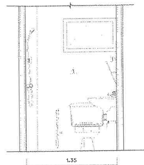
รูปตัด A มาตราส่วน 1:25
