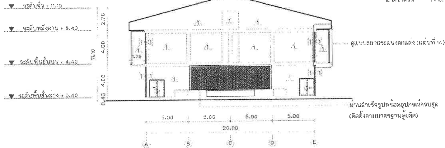
รูปตัด A ที่ปรับปรุง มาตราส่วน 1:200
