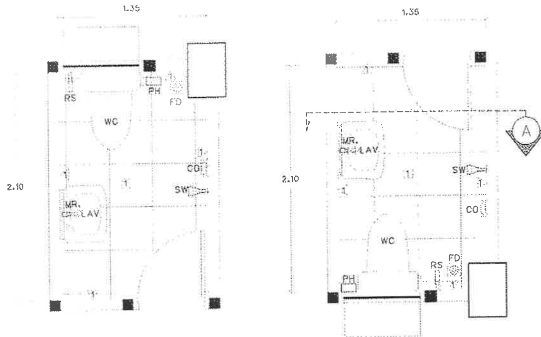
แบบขยายห้องน้ำ มาตราส่วน 1:25
