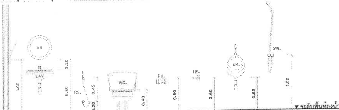
แบบขยายห้องน้ำ มาตราส่วน 1:25
