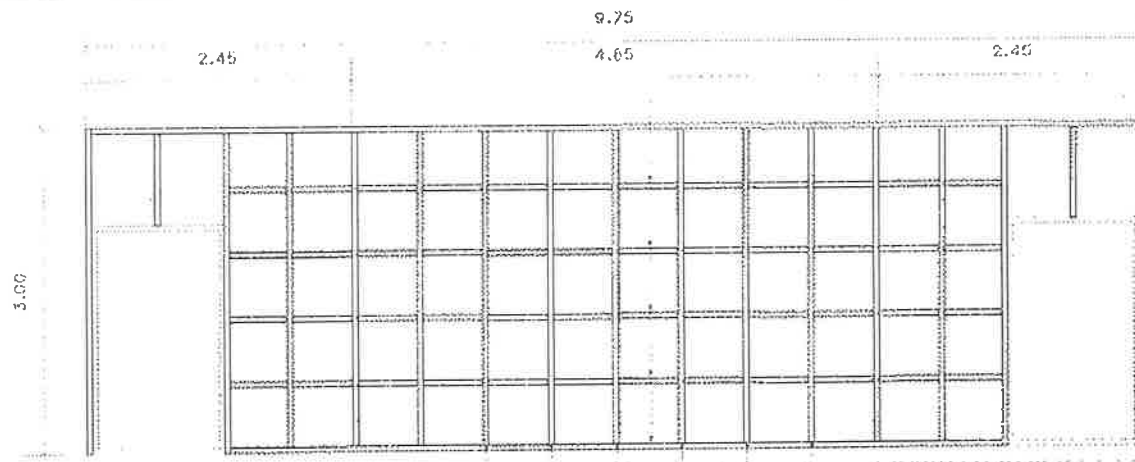
ขยายโครงสร้างผนังสำเร็จรูป (เวที) มาตราส่วน 1:50
