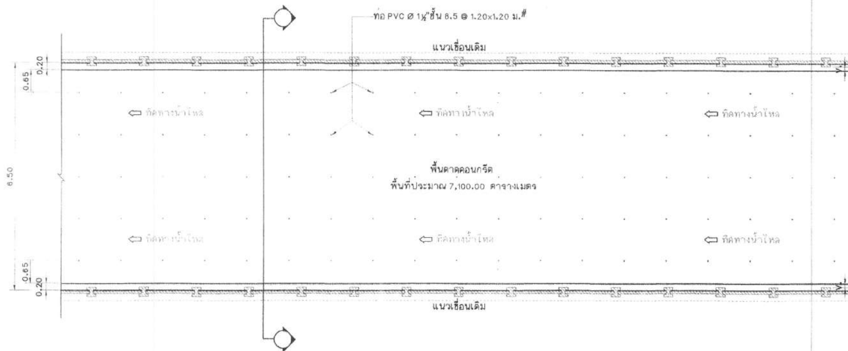
แบบขยายแปลนพื้นดาดคอนกรีต (ช่วงความกว้าง 6.50 ม.) มาตรฐาน 1:75
