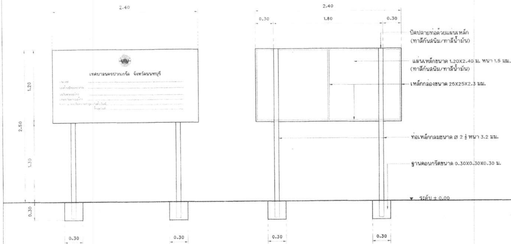
รูปด้านหน้าป้ายโครงการ มาตราส่วน 1:25
