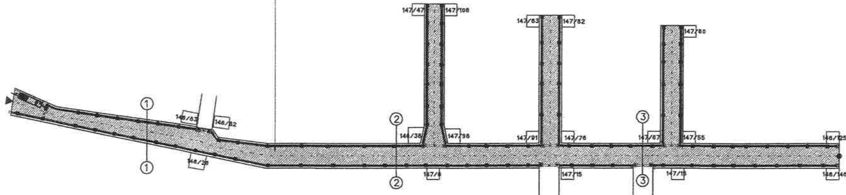
ผังบริเวณการก่อสร้างปรับปรุงถนน และวางท่อระบายน้ำ มาตราส่วน 1:1000
