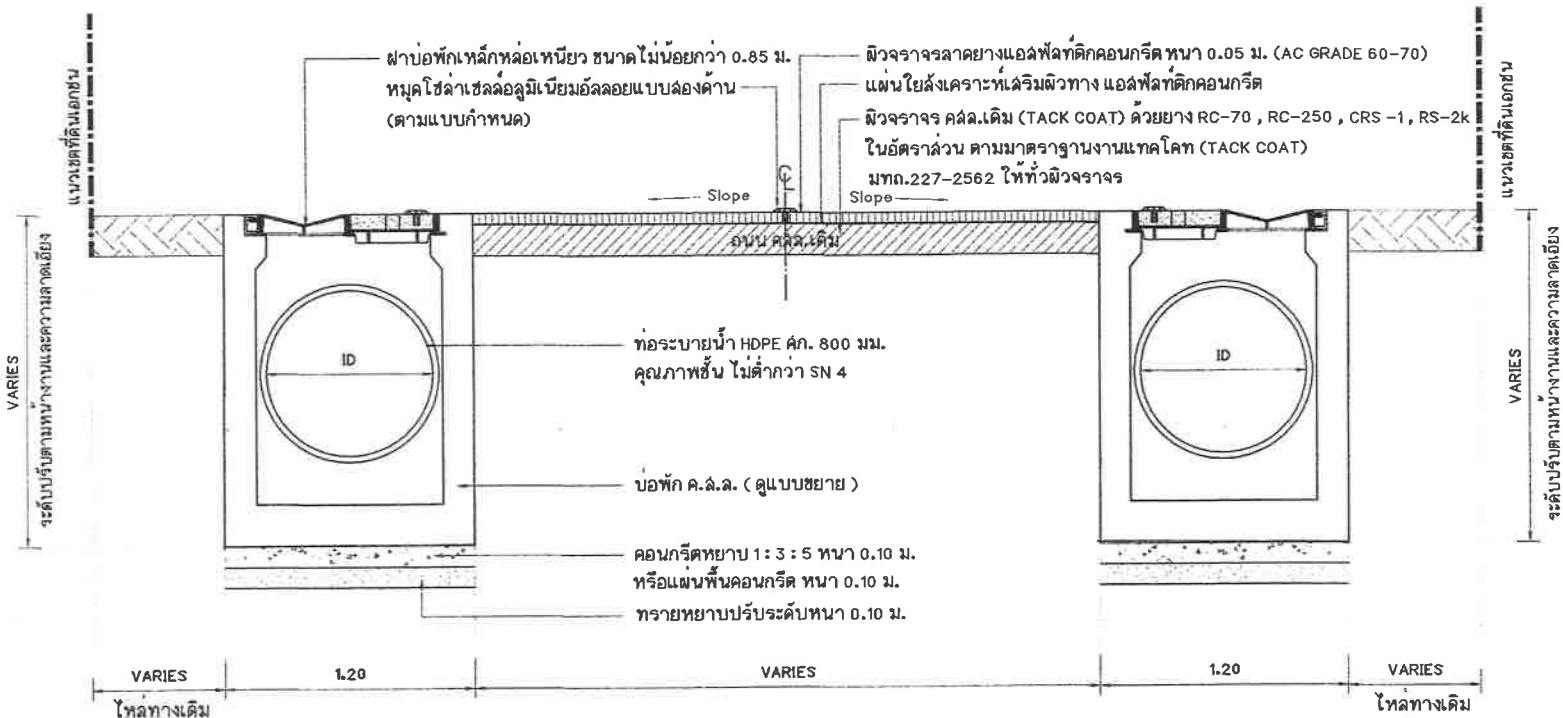
แบบขยายรูปตัด 2 (ถนนเมน) มาตราส่วน 1:25
