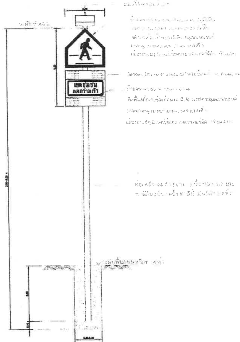
แบบที่ 6 ป้ายเตือนเขตชุมชนลดความเร็ว ไฟกระพริบโซล่าเซลล์
