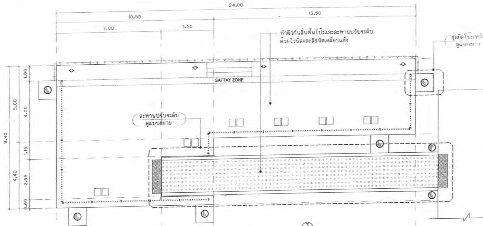
แบบแปลนโป๊ะทำเทียบเรือโดยสาร
