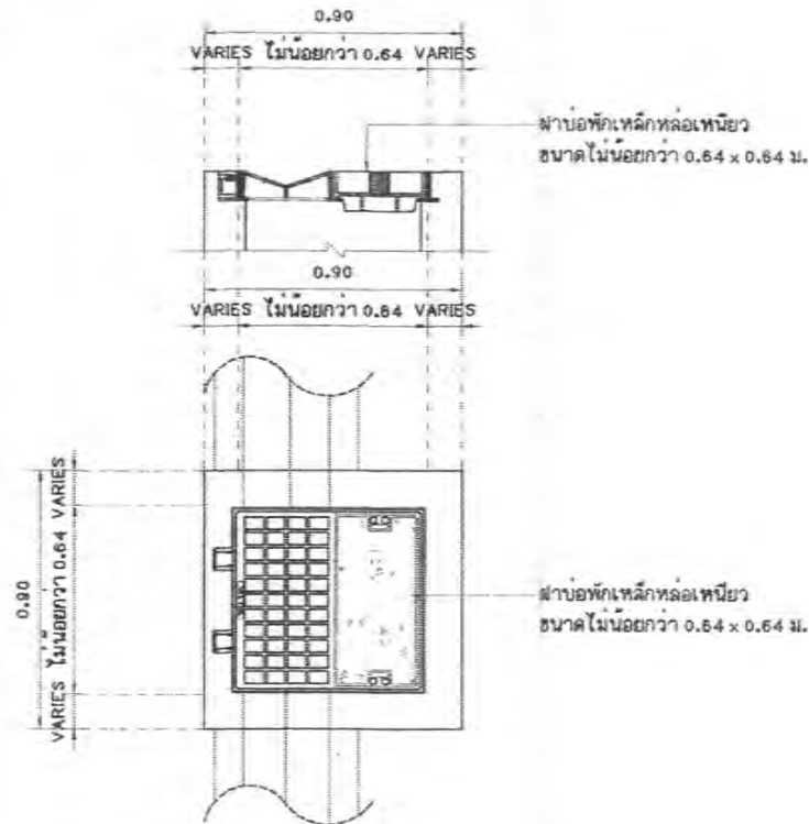
แบบขยายผ้าบอพักเหล็กหล่อเหนียว 1
