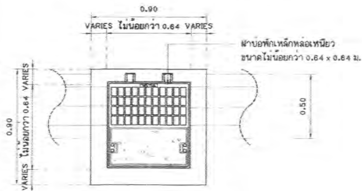
แบบขยายแปลนรางวี
