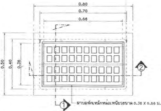
แบบขยายฝาบ่อพักรางวีเหล็กหล่อเหลี่ยม มาตราส่วน 1 : 10
