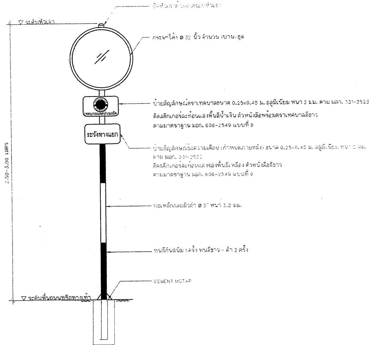
รูปด้านหน้าแบบกระจกโค้ง แบบการติดตั้งกระจกโค้ง แบบฐานรากที่ 1
