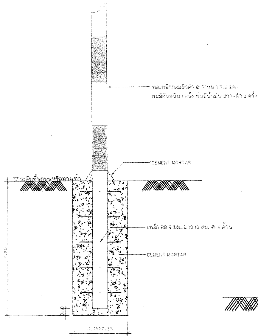
แบบขยายฐานจาก ①
