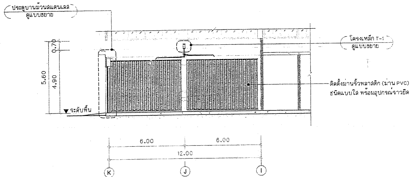
รูปตัด-B (ระบบล่างรถ) SCALE 1:125
