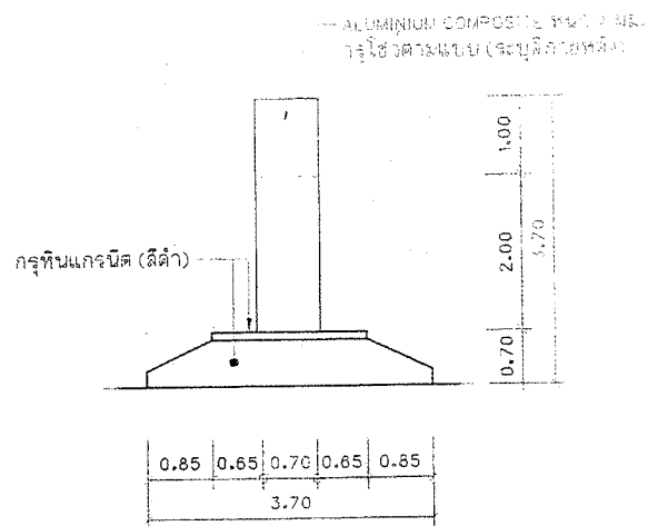
รูปด้าน-2 (ป้ายชื่ออาคาร) SCALE 1:75
