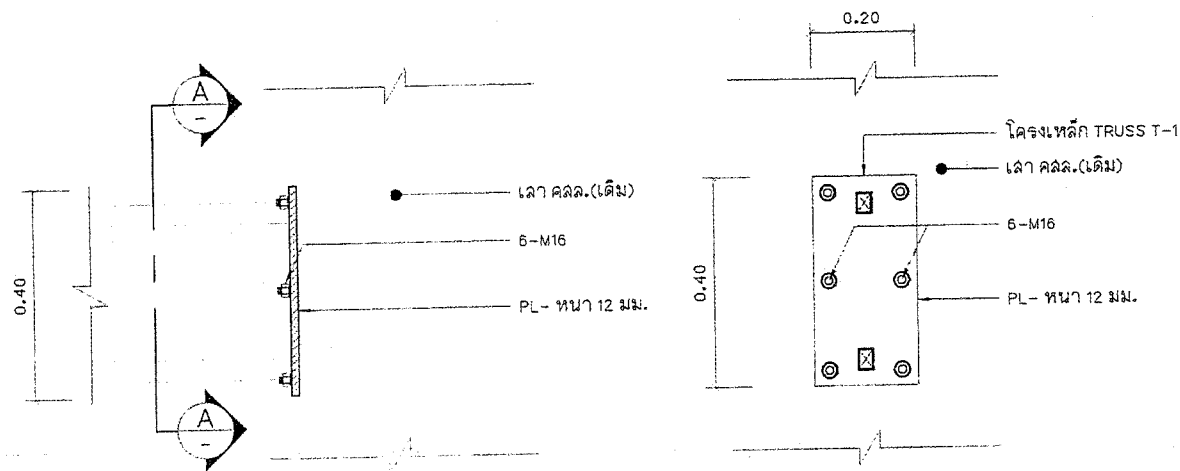
แบบขยายการติดตั้ง SCALE 1:10
