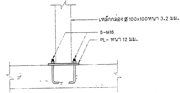
แบบขยายการติดตั้งเสาปายี่้ออาคาร SCALE 1:10
