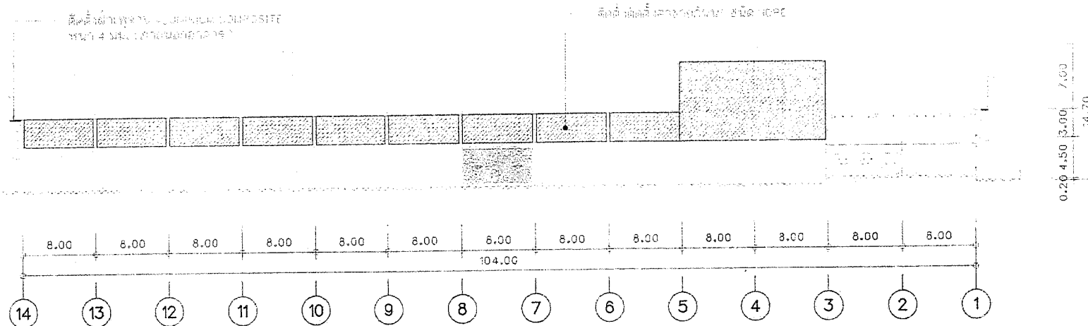
รูปตัด-A (ติดตั้งดาดฟ้ากันชน HDPE)
