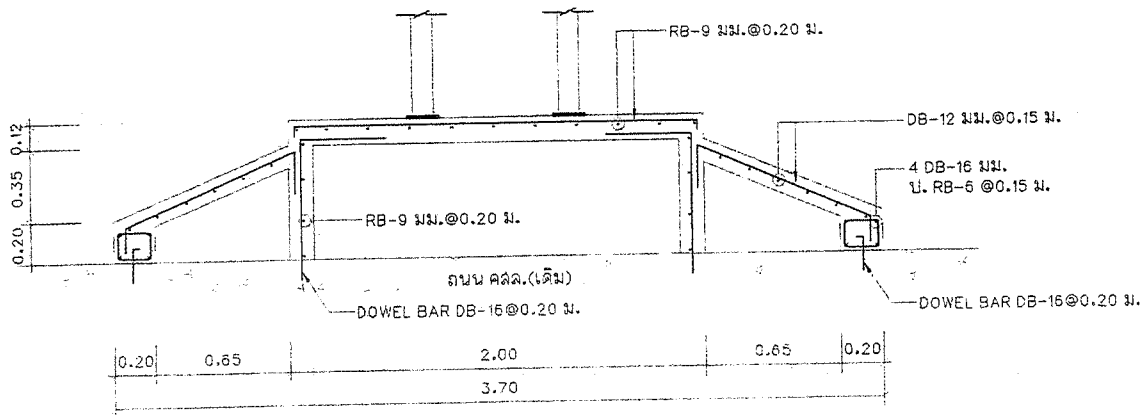
แบบขยายฐานราก (ปายี่้ออาคาร) SCALE 1:25
