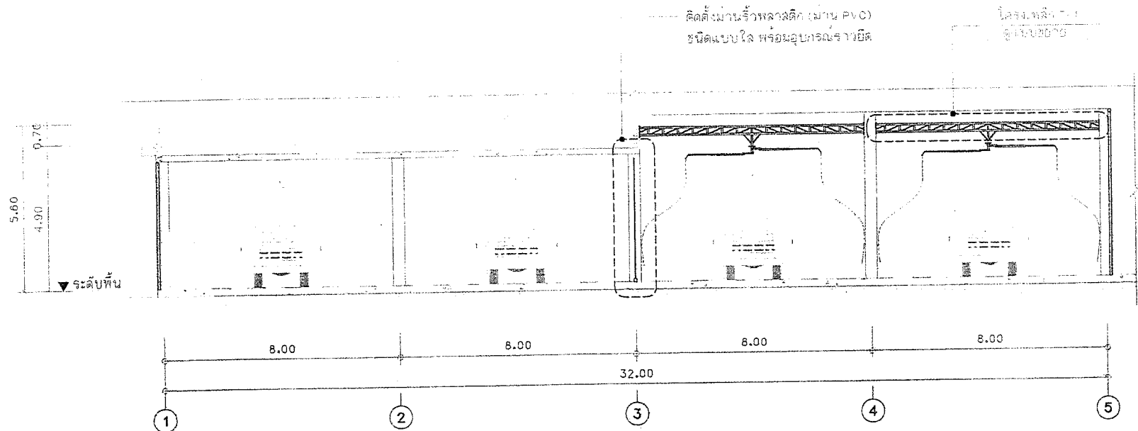
รูปตัด-A (ระบบล่างรถ) SCALE 1:125
