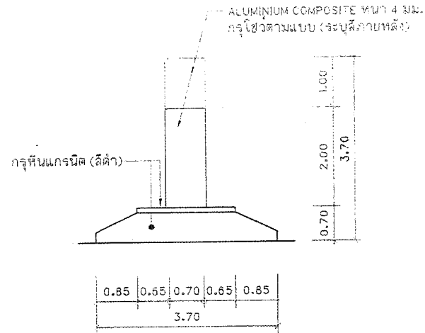
รูปด้าน-4 (ป้ายชื่ออาคาร) SCALE 1:75
