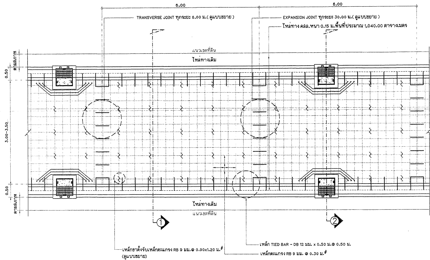
แปลนการวางเหล็กตะแกรงและรอยต่อถนน คลล. มาตราส่วน 1 : 50
