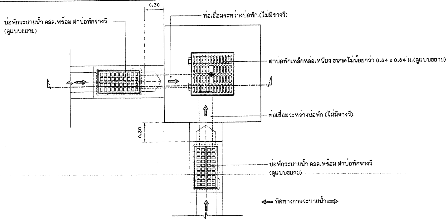
แปลนขยายช่องเปิดรับน้ำบ่อกัก(หัวมุม)
