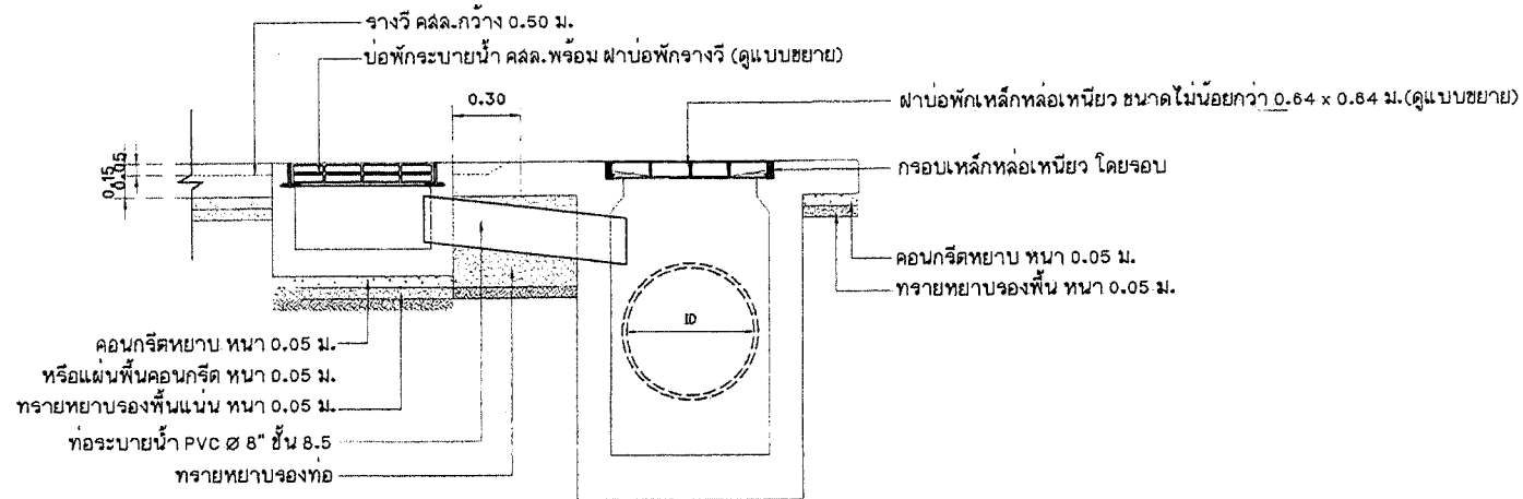
แบบขยายรูปตัดการเชื่อมต่อท่อ บ่อกัก(หัวมุม)
