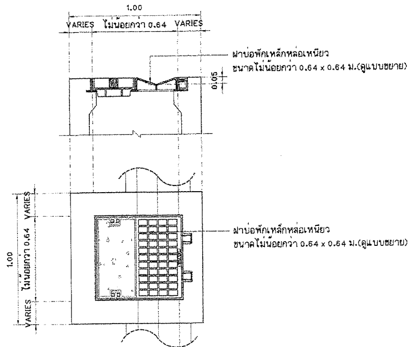
แบบขยายฝาป้องกันเหล็กหล่อเหนียว 1 มาตราส่วน 1:20
