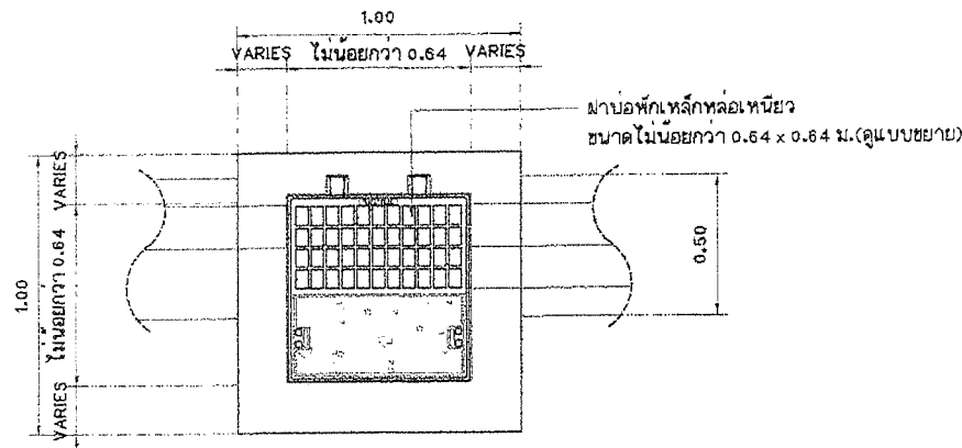
แบบขยายฝาป้องกันเหล็กหล่อเหนียว 1 มาตราส่วน 1:20
