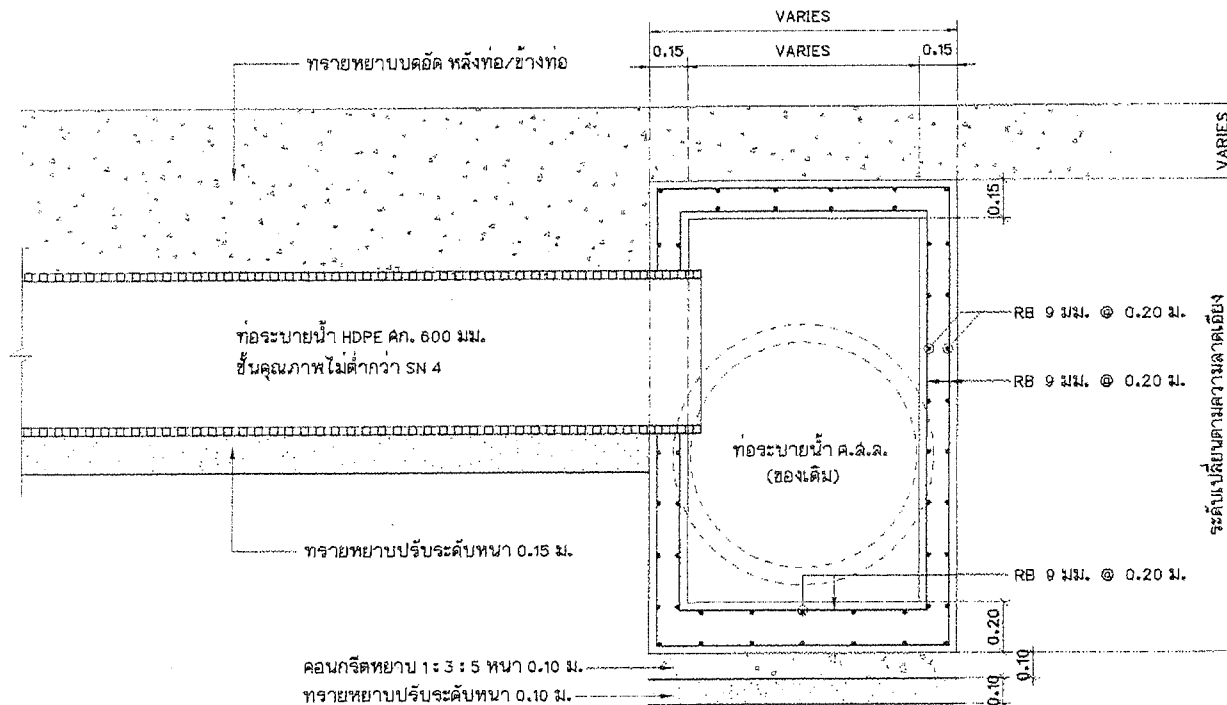
แปลนการเชื่อมต่อในกรณีเชื่อมกับท่อระบายน้ำช่องเดิม มาตราส่วน 1:20
