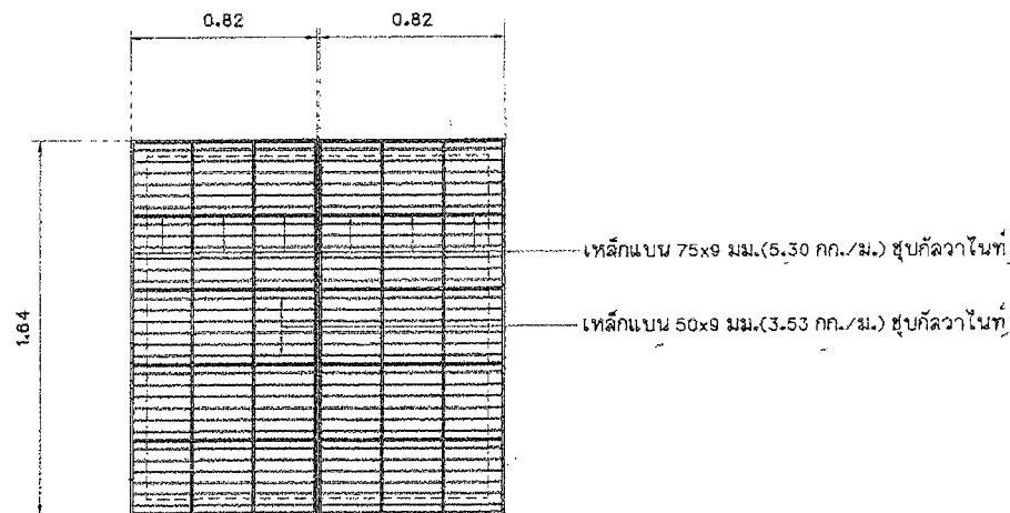
แปลนขยายฝาตะแกรงเหล็กบ่อพัก คลล.1
