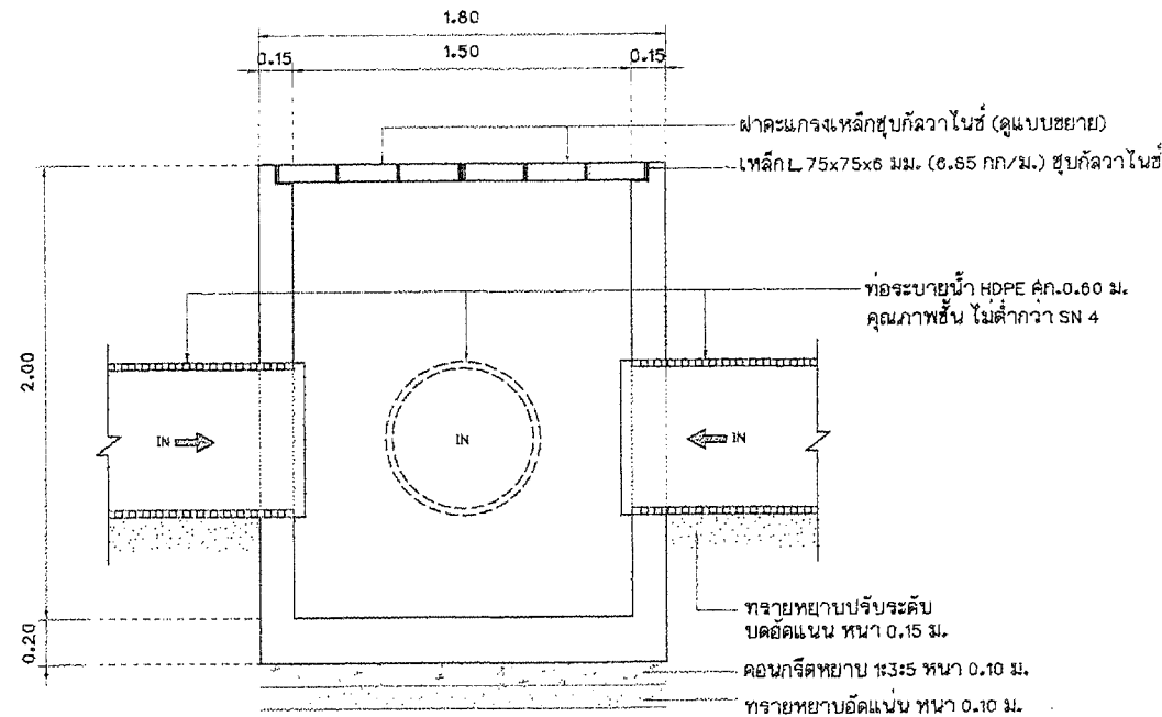
ขยายรูปตัดบ่อพัก คลล.1
