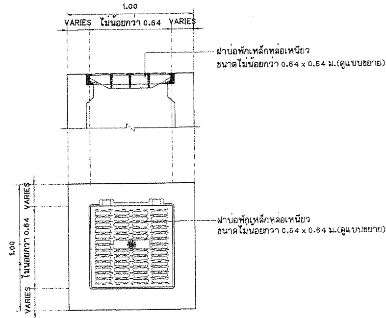
แบบขยายฝาป้องกันเหล็กหล่อเหนียว 2 มาตราส่วน 1:20
