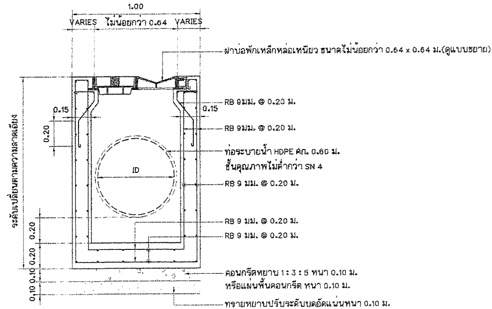
แบบขยายรูปตัดโครงสร้างบ่อพัก ค.ล.ล มาตราส่วน 1:20
