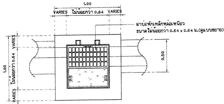
แบบขยายฝาบ่อพักเหล็กหล่อเหนียว 1 มาตราส่วน 1:20
