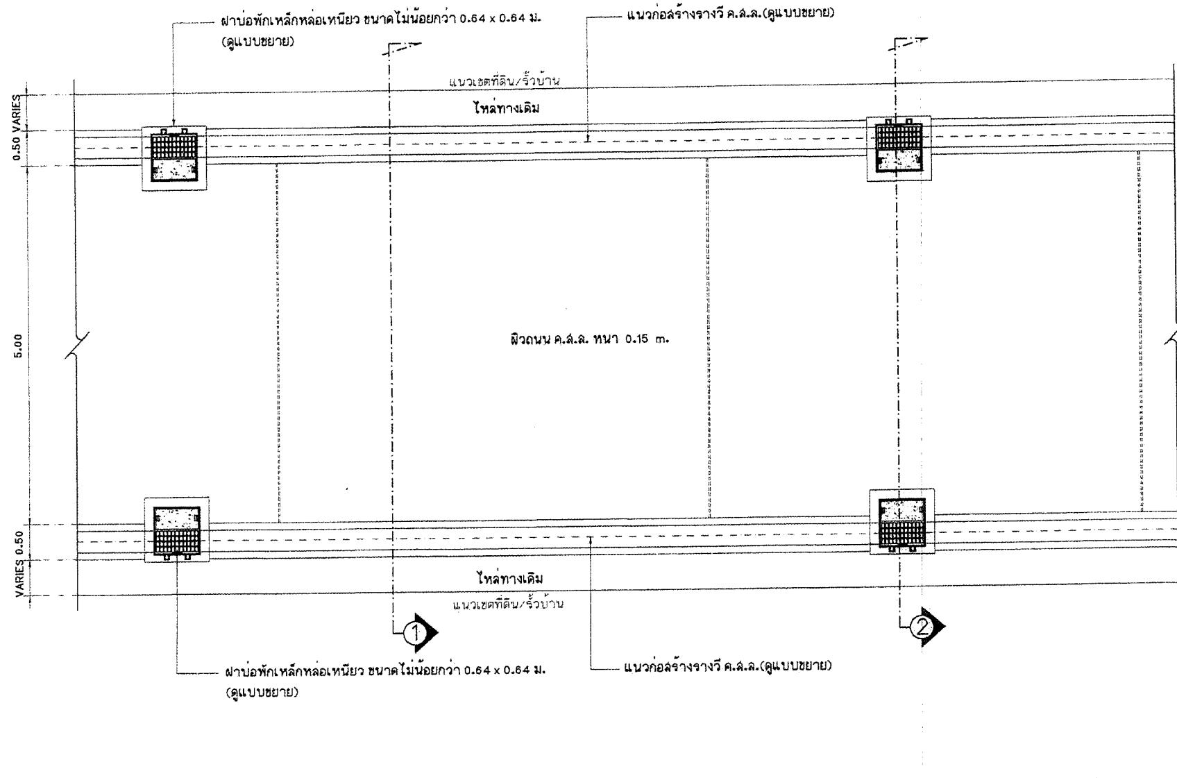
แปลนถนน และการวางบ่อพัก คลล. มาตราส่วน 1 : 50
