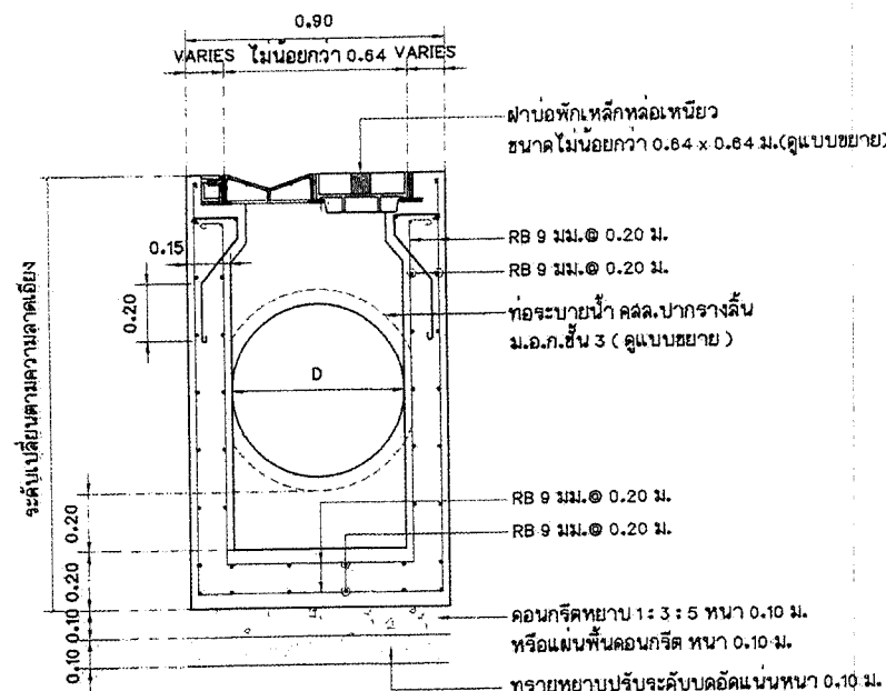
แบบขยายบ่อพัก คลล์. มาตรา ๖๖ 1:20
