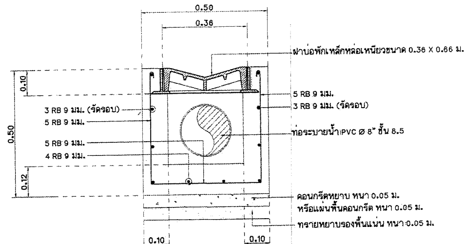
แบบขยายรูปตัด ① บ่อพักระบายน้ำ คล. พร้อม ฝาบ่อพักรางวิ
