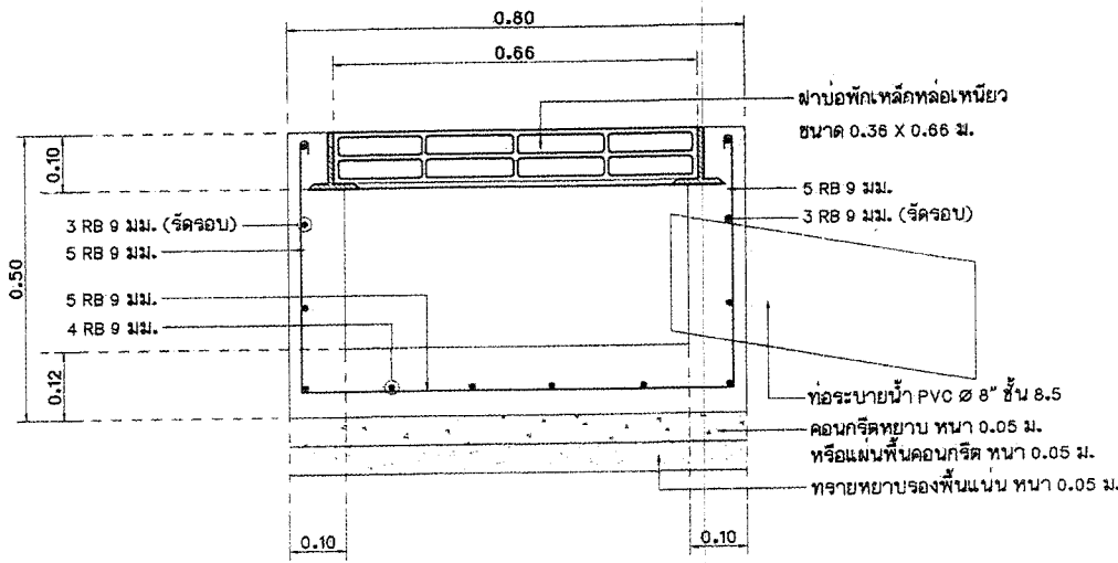
แบบขยายรูปตัด ② บ่อพักระบายน้ำ คล. พร้อม ฝาบ่อพักรางวิ
