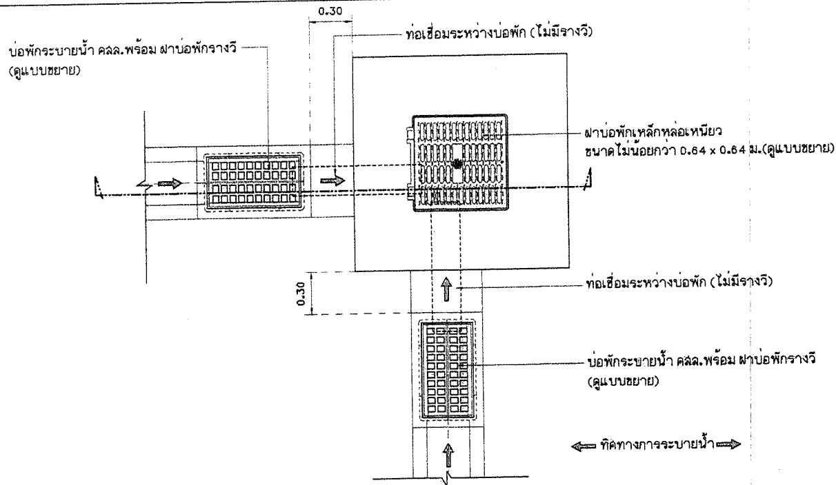
แปลนขยายช่องเปิดรับน้ำบ่อพัก(หัวมุม)
