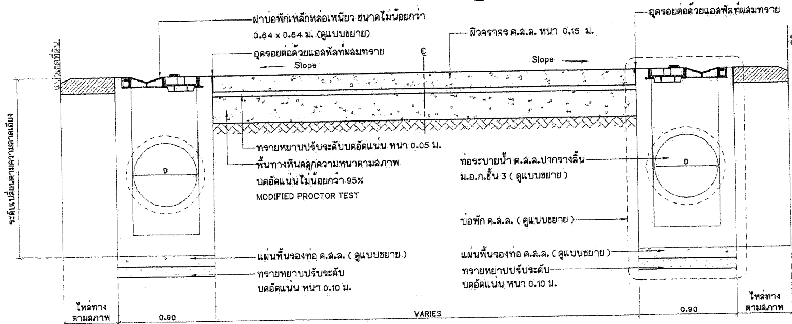
รูปตัด มาตราส่วน 1 : 25
