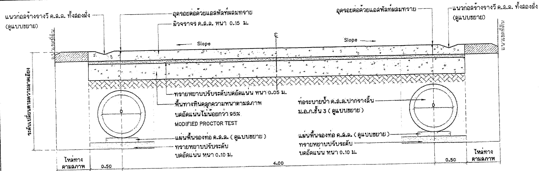
รูปตัด มาตราส่วน 1 : 25
