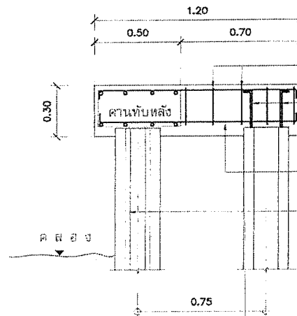
รูปตัด (กรณีไม่มีทางเท้า) มาตราส่วน 1 : 20
