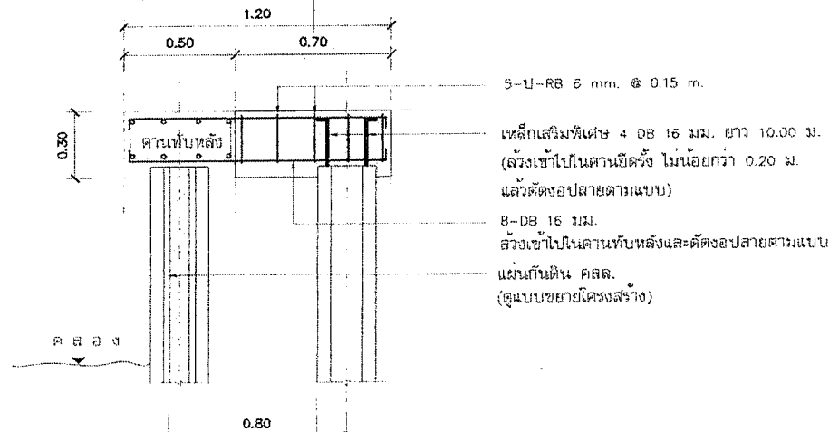
รูปตัด (กรณีมีทางเท้า) A มาตราส่วน 1:20
