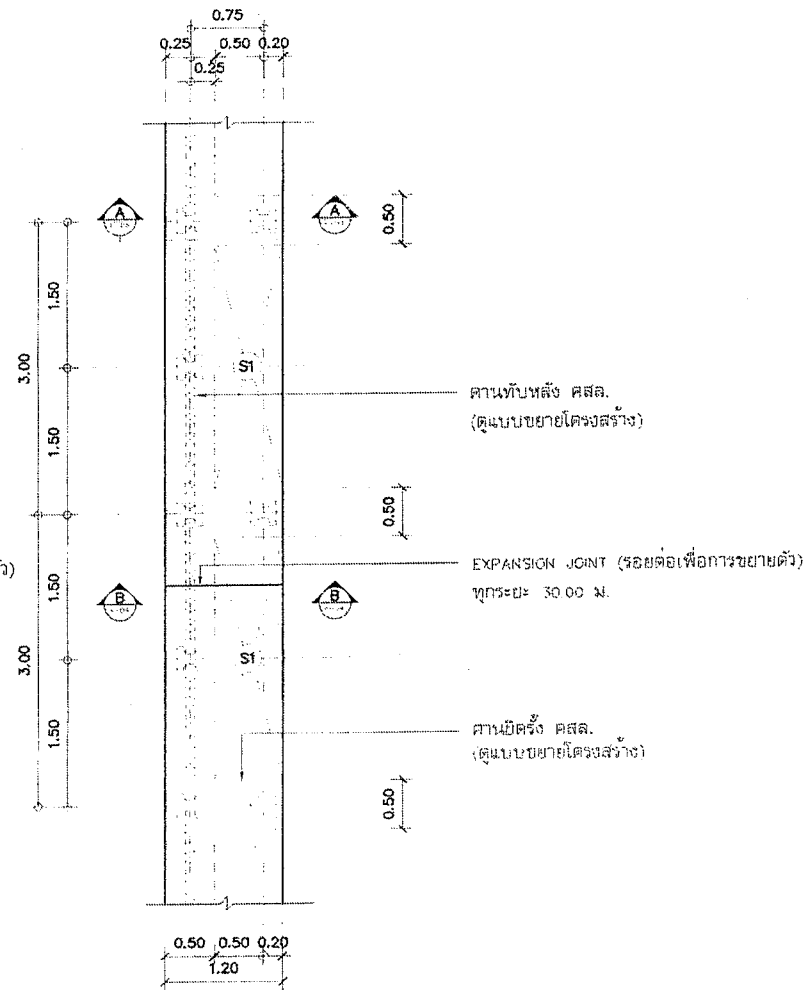
แปลนเสาเข็ม, คาน, พื้น คสล. (กรณีมีทางเท้า คสล.) มาตราส่วน 1 : 50
