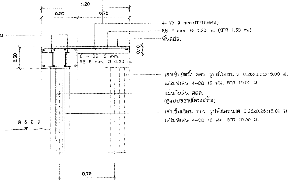
รูปตัด (กรณีมีทางเท้า) B มาตราส่วน 1:20
