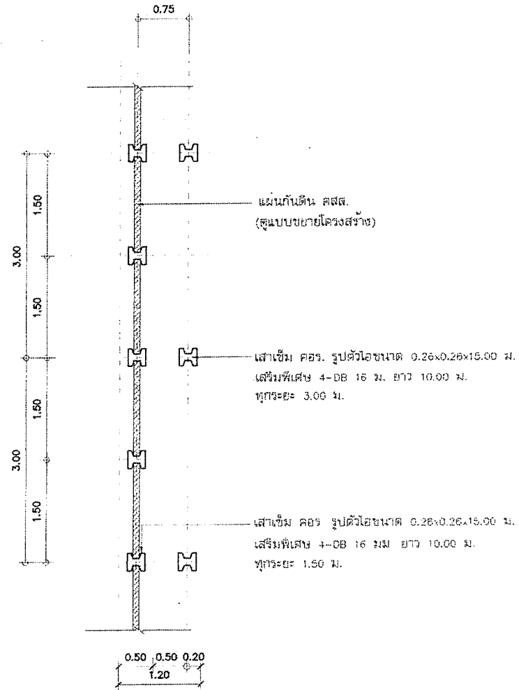
แปลนเสาเข็ม, กำแพงกันดิน (กรณีไม่มีทางเท้า คสล.)
