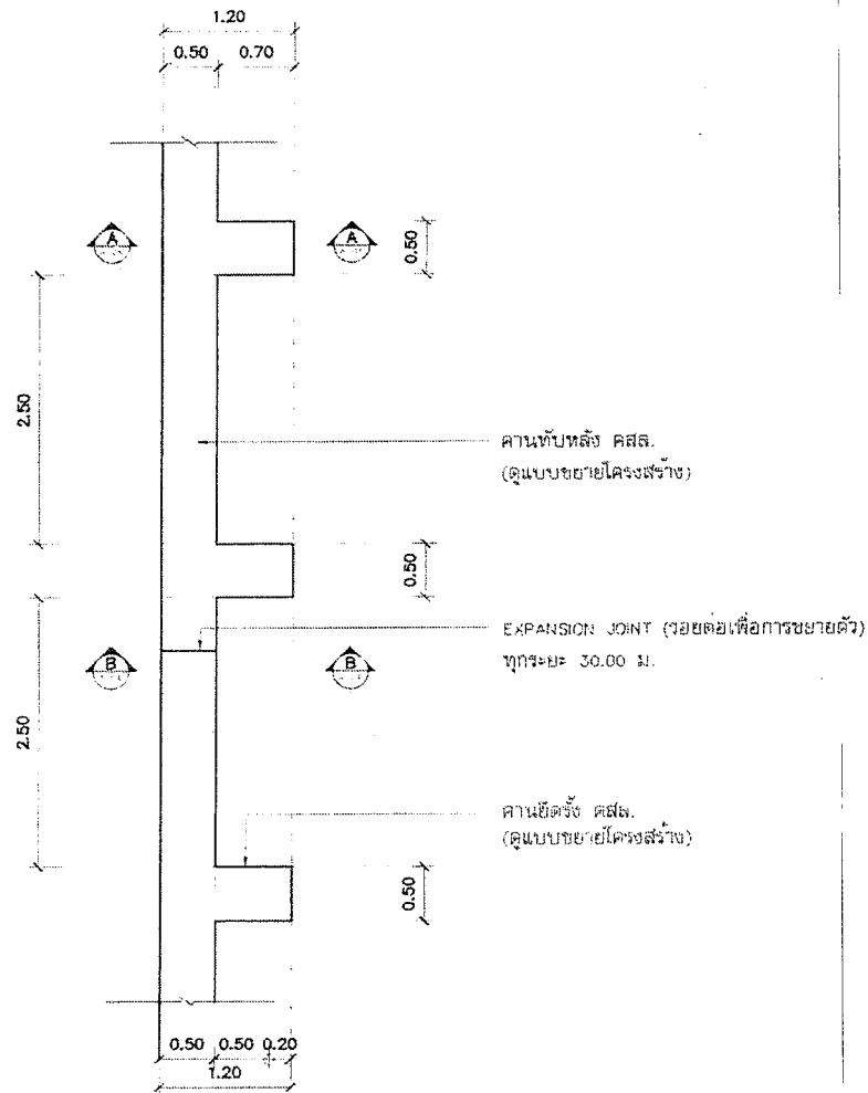
แปลนเขื่อน คสล.
