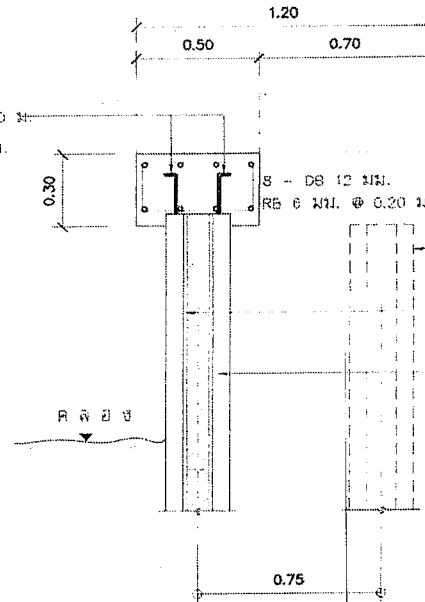
รูปตัด (กรณีไม่มีทางเท้า) มาตราส่วน 1 : 20
