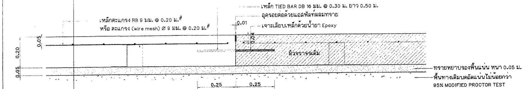
แบบขยาย LONGITUDINAL JOINT ระหว่างผิวจราจรเดิมกับผิวจราจรใหม่ c/l มาตราส่วน 1:10
