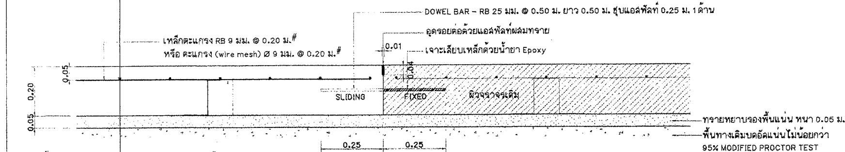
แบบขยาย TRANSVERSE JOINT ระหว่างผิวจราจรเดิมกับผิวจราจรใหม่ ทุกระยะ 6.00 ม. มาตราส่วน 1:10
