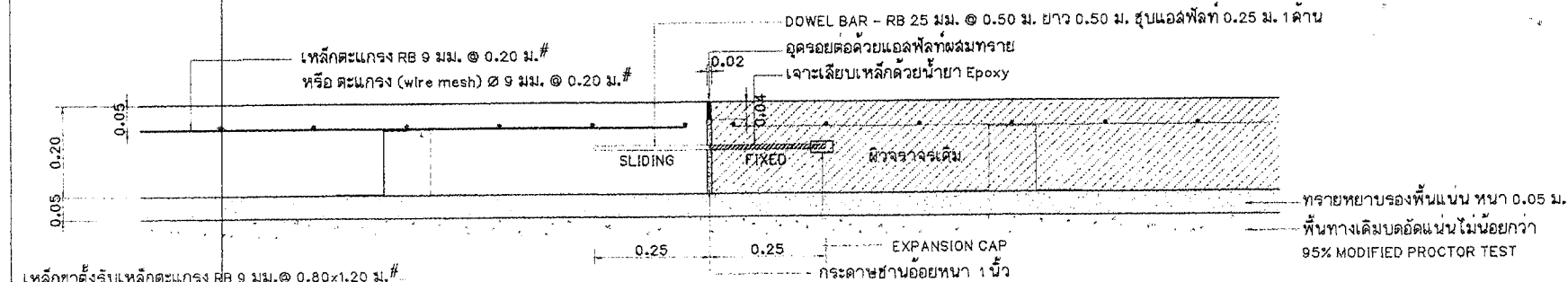
แบบขยาย EXPANSION JOINT ระหว่างผิวจราจรเดิมกับผิวจราจรใหม่ ทุกระยะ 30.00 ม. มาตราส่วน 1:10
